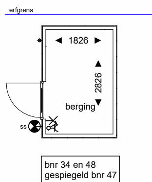
Begane grond
