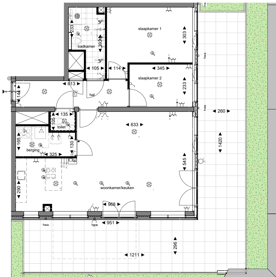
4e verdieping
