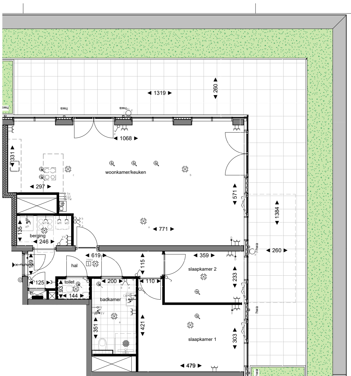
4e verdieping
