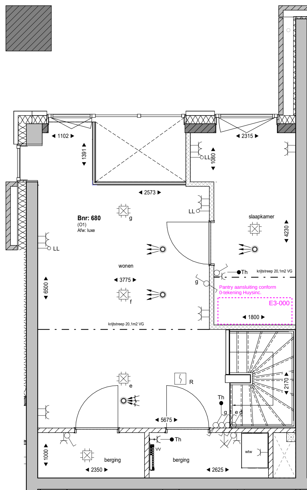
Verdieping
