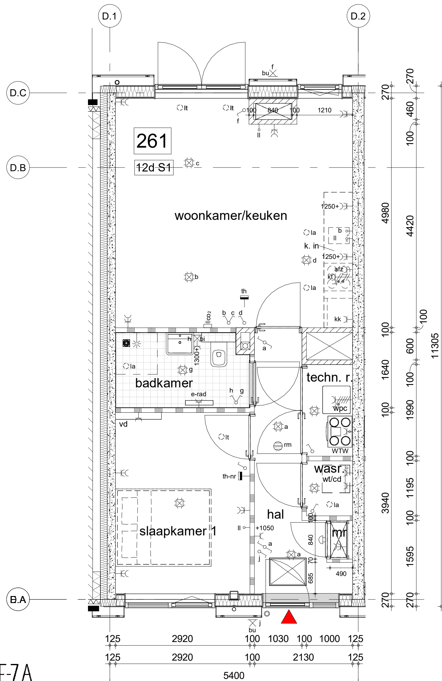
begane grond
