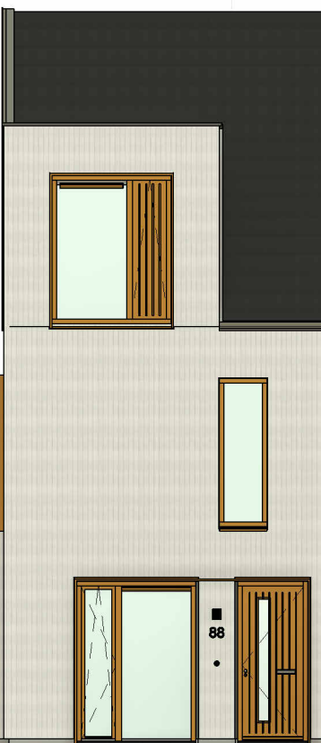
Rechter zijgevel optie uitbouw 1,8m / 2,4m
