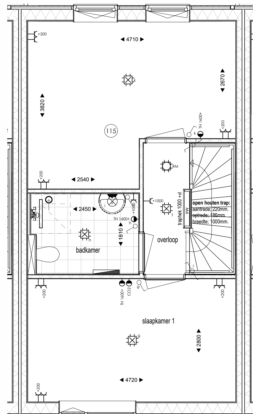
Eerste verdieping optie slaapkamer samenvoegen
