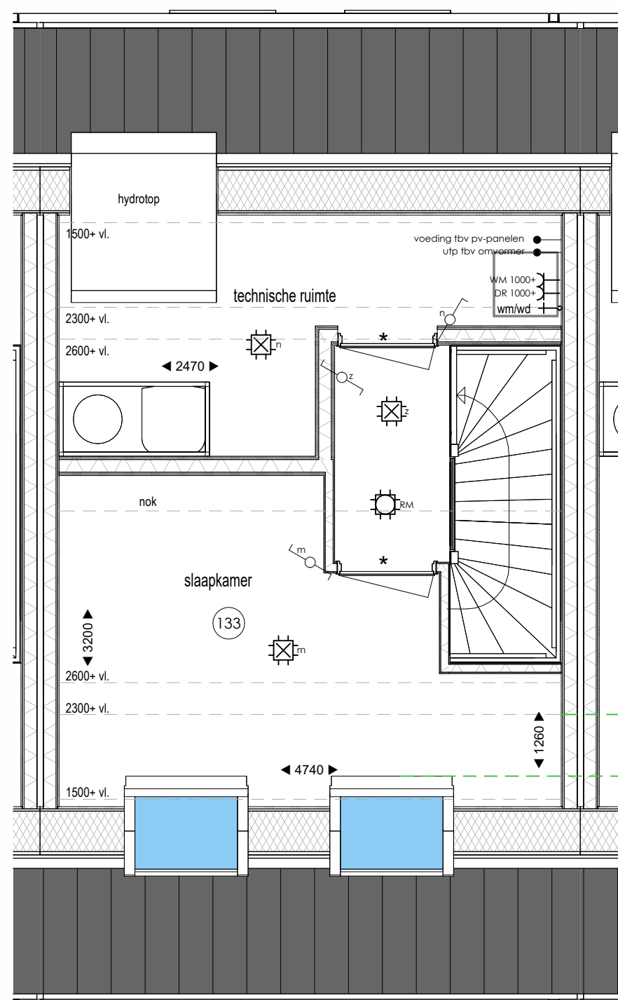
Tweede verdieping optie extra ruimte
