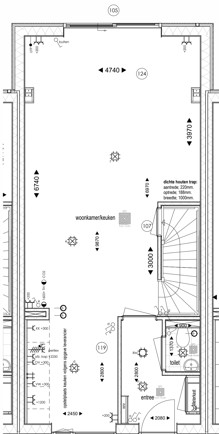
Begane grond optie uitbouw 1,8m + trapkast
