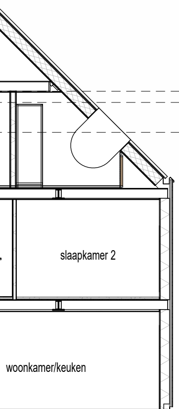
Doorsnede optie slaapkamer zolder + afwerking
