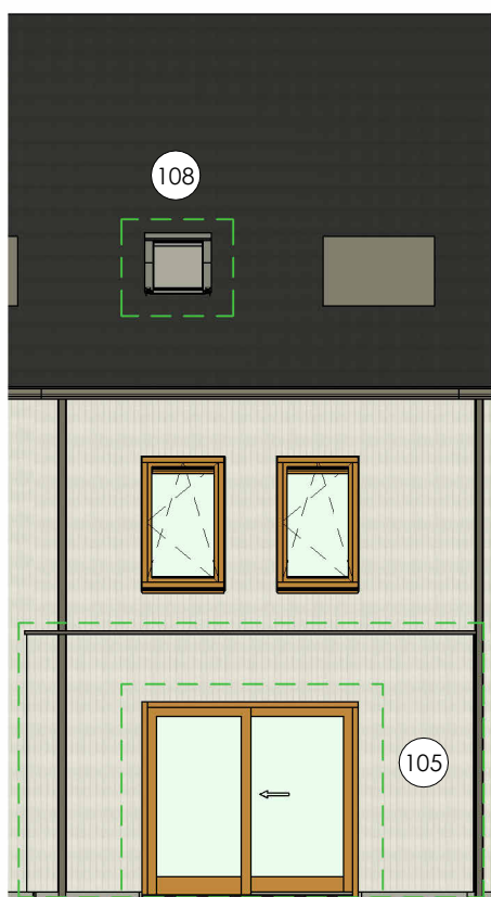
Achtergevel optie uitbouw 1,8m / 2,4m + dakraam + schuifpui
