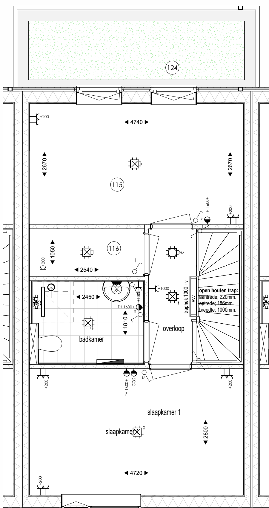
Eerste verdieping optie uitbouw 1,8m + slaapkamer samenvoegen met bergruimte
