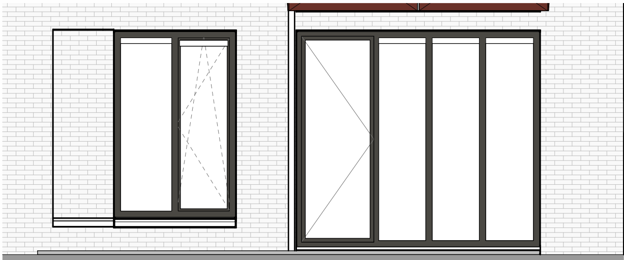
Gevelfragment Noordwestgevel 1:50
