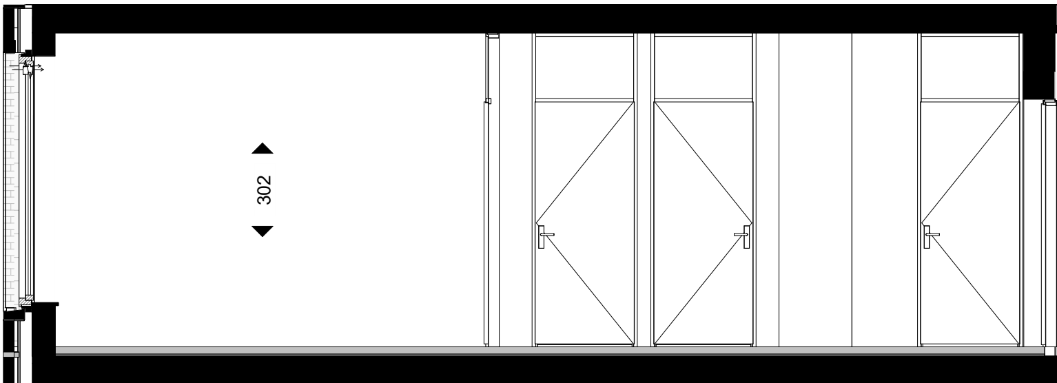
Lengtedoorsnede 1:50
