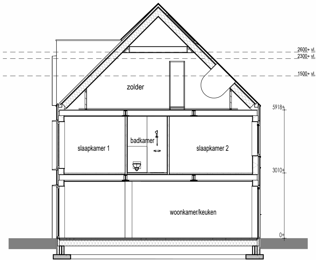
Doorsnede 1 : 100
