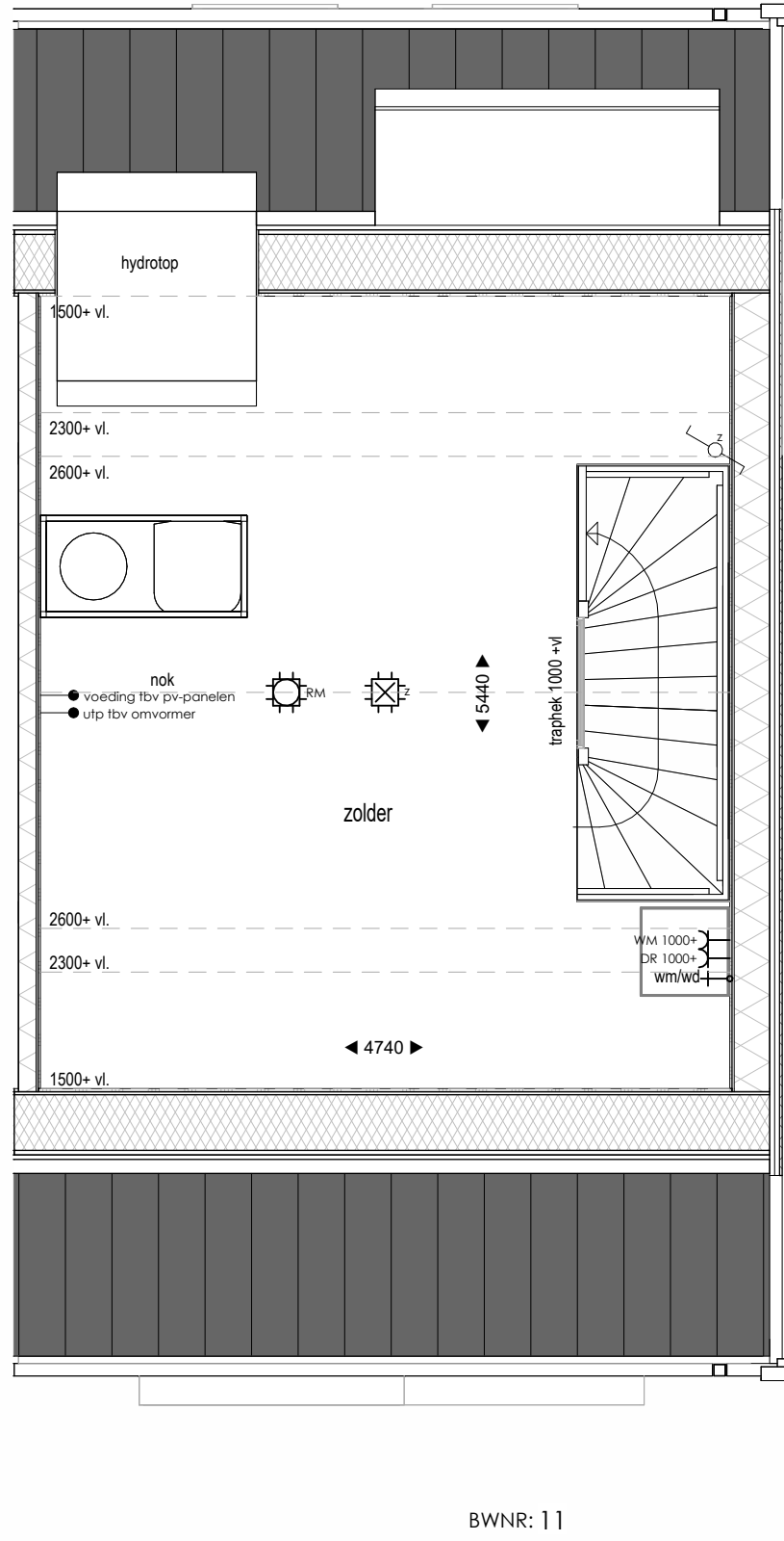
Tweede verdieping 1 : 50
