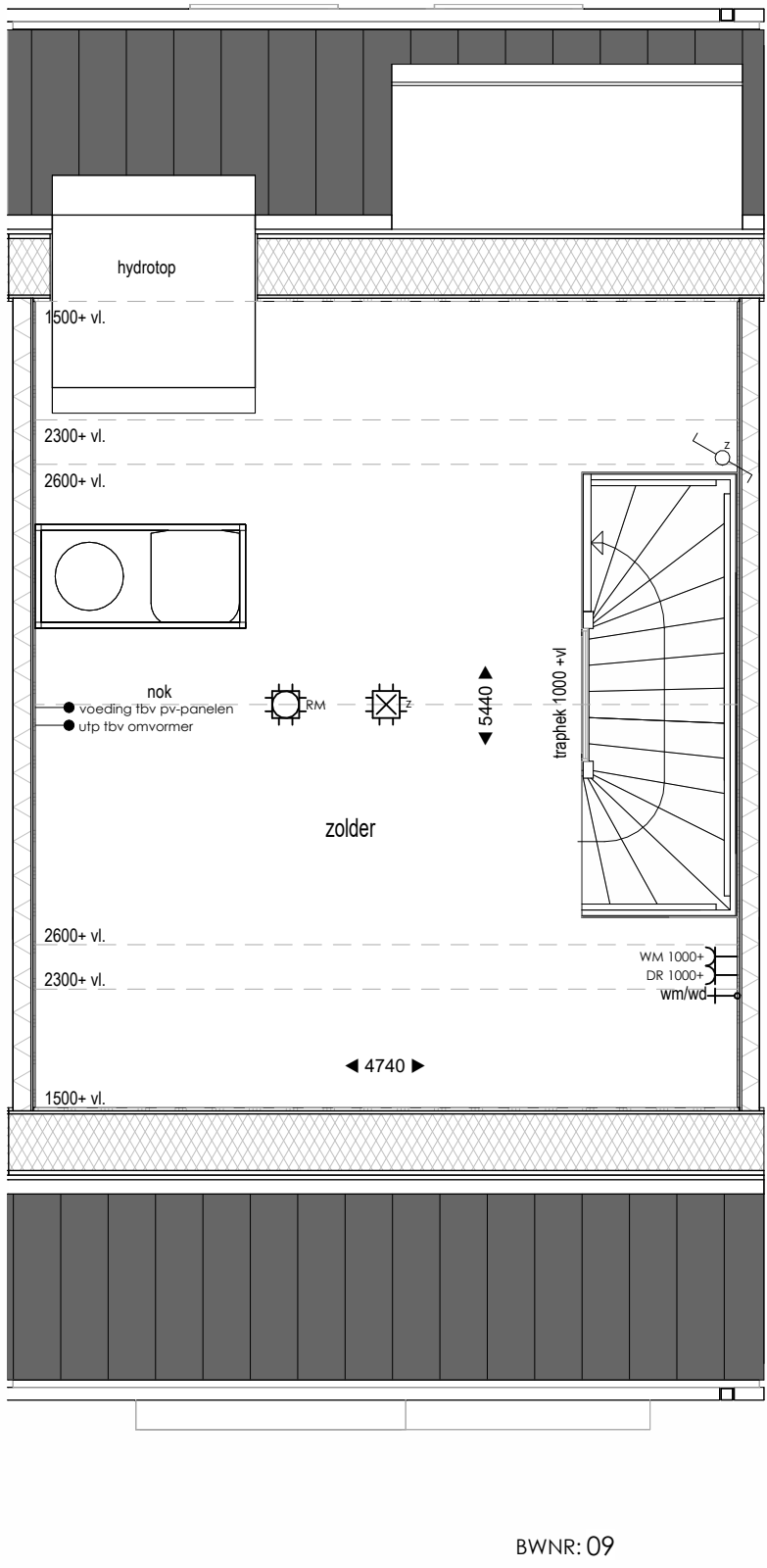
Tweede verdieping 1 : 50
