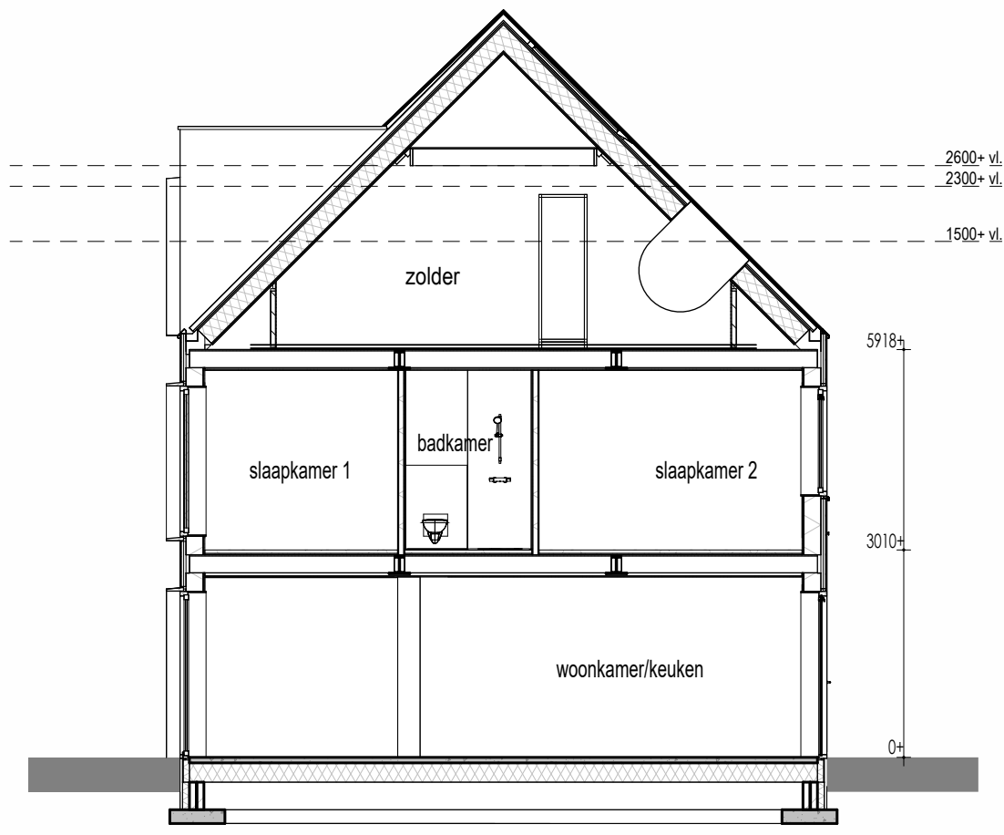
Doorsnede 1 : 100
