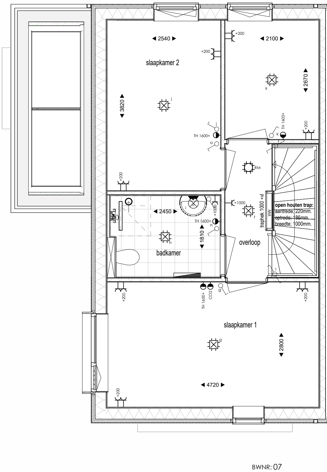
Eerste verdieping 1 : 50
