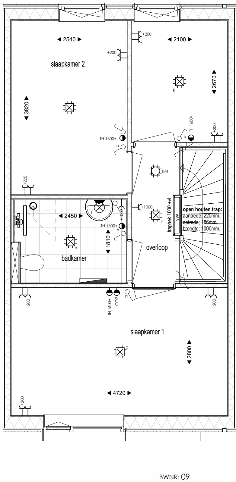
Eerste verdieping 1 : 50
