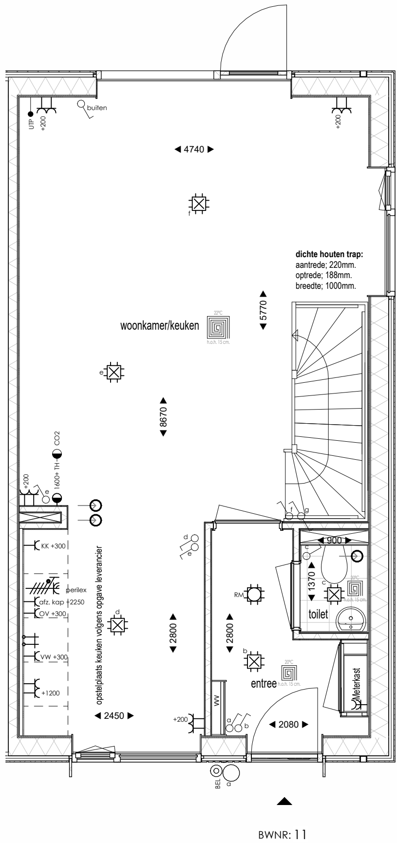
Begane grond 1 : 50
