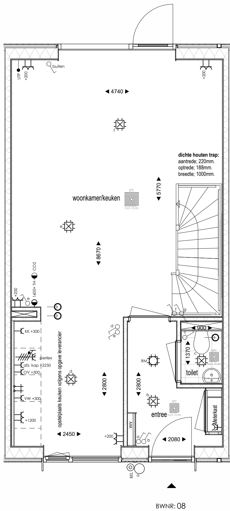
Begane grond 1 : 50
