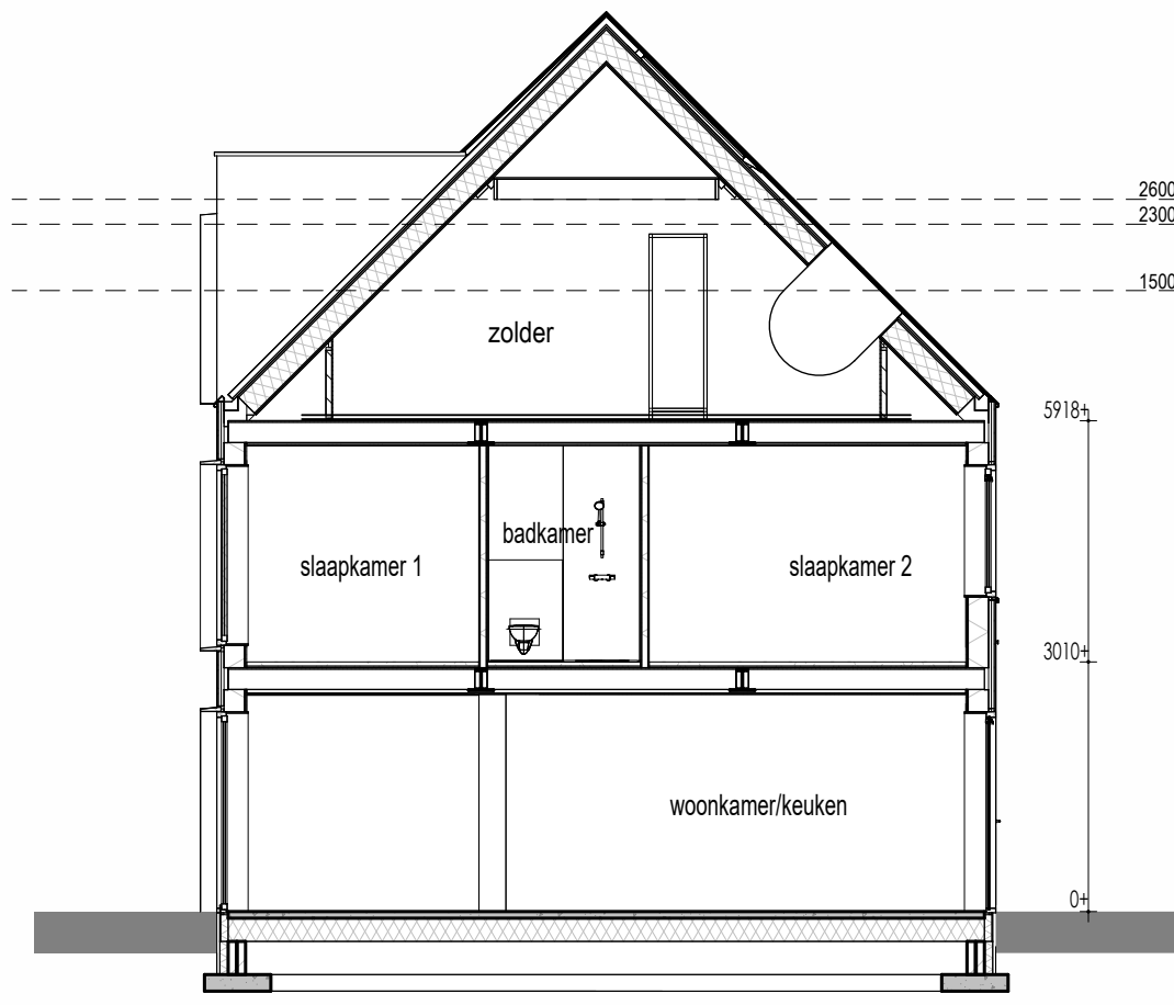
Doorsnede B 1 : 100
