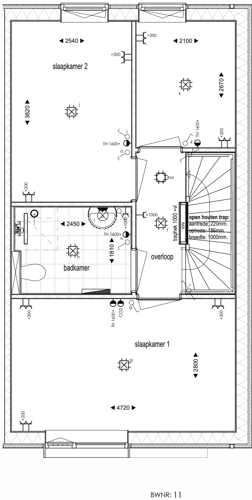
Eerste verdieping 1 : 50
