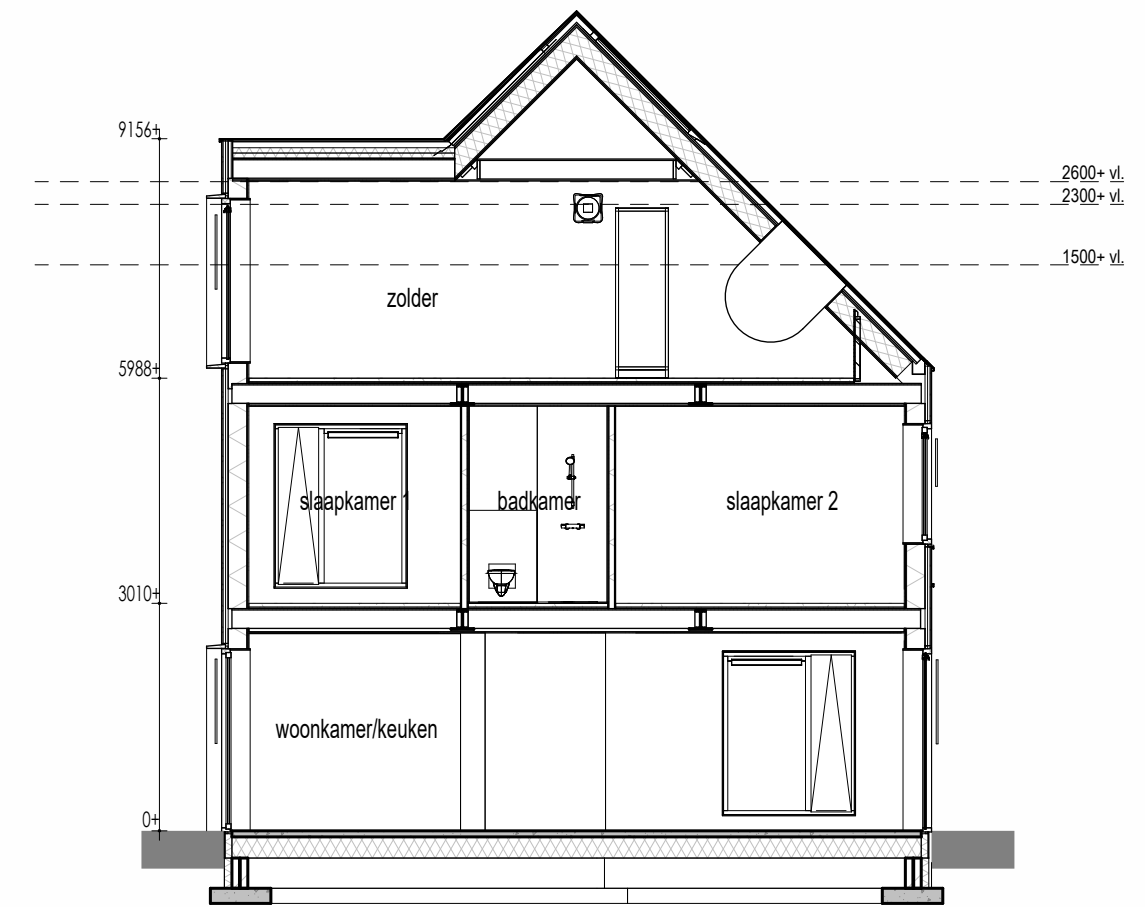
Doorsnede 1 : 100
