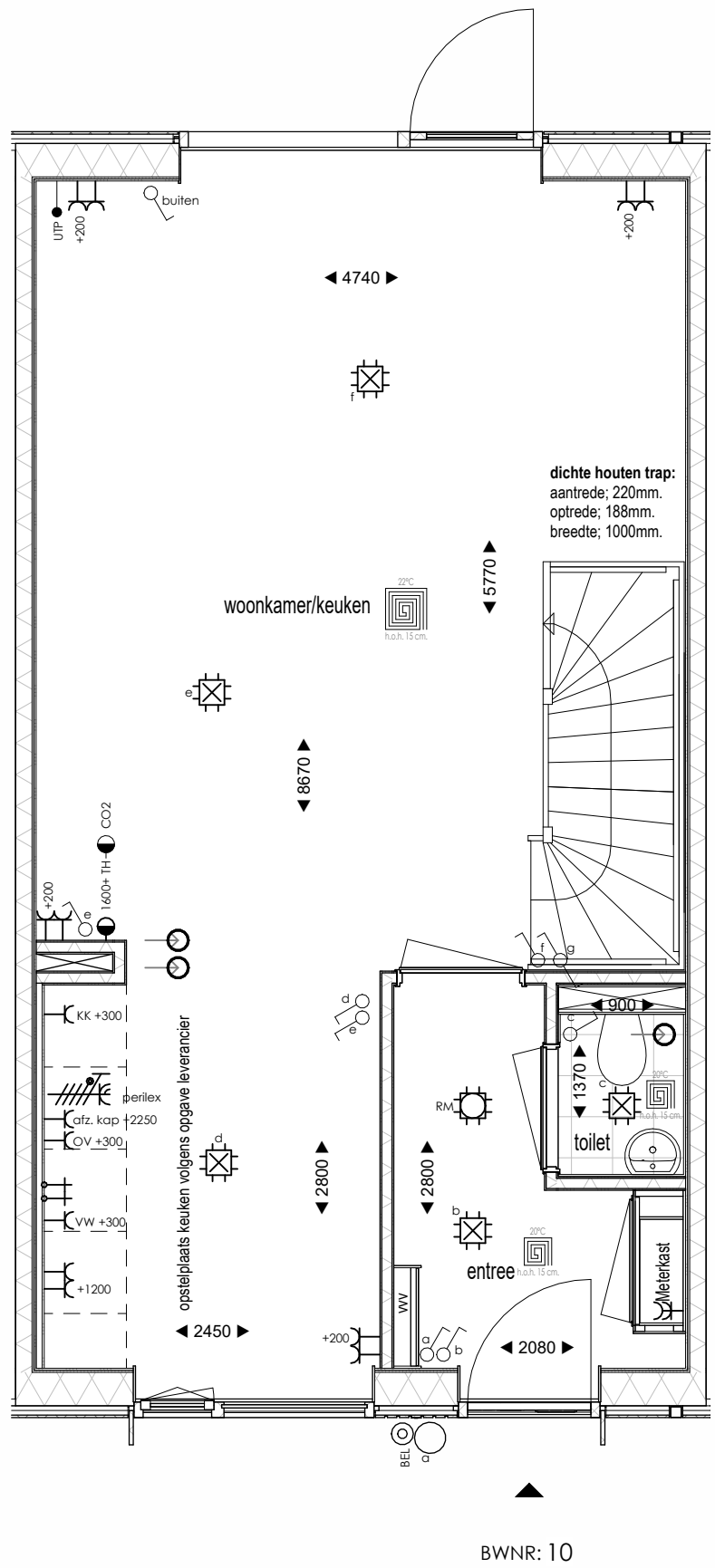
Begane grond 1 : 50
