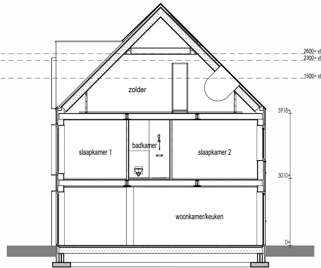
Doorsnede 1 : 100
