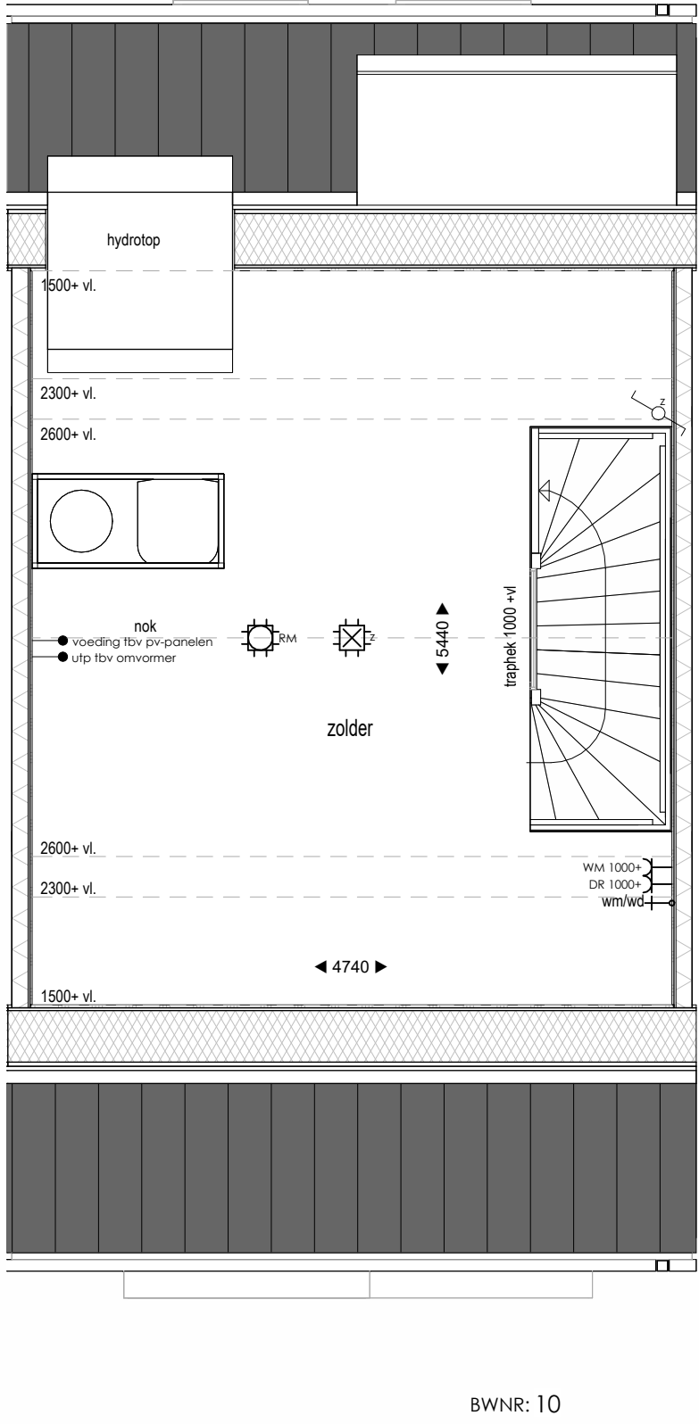
Tweede verdieping 1 : 50
