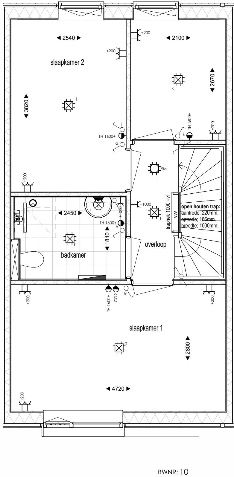
Eerste verdieping 1 : 50
