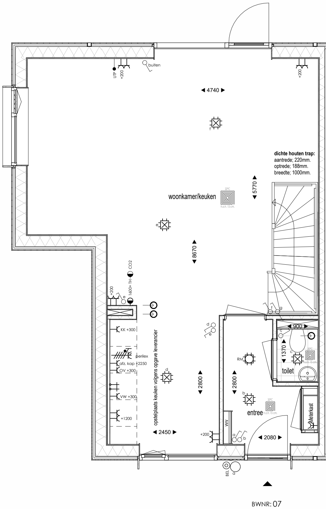
Begane grond 1 : 50
