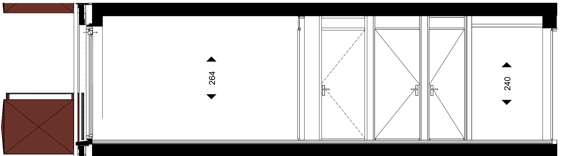
Lengtedoorsnede 1:50
