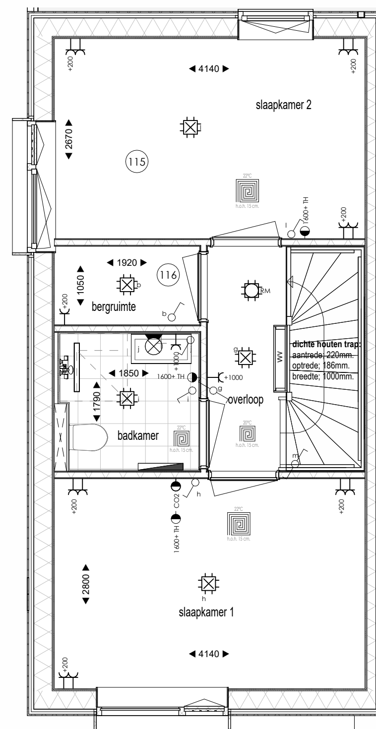
Eerste verdieping optie slaapkamer samenvoegen met bergruimte
