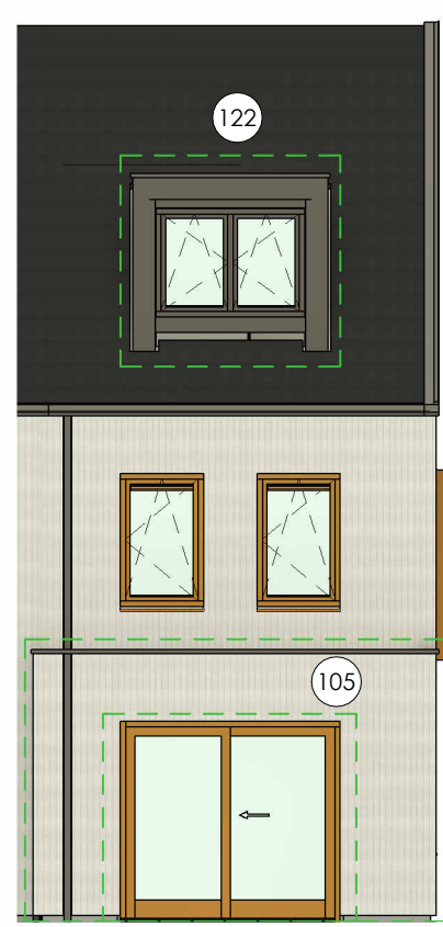
Achtergevel optie uitbouw 1,8m / 2,4m + dakkapel + schuifpui
