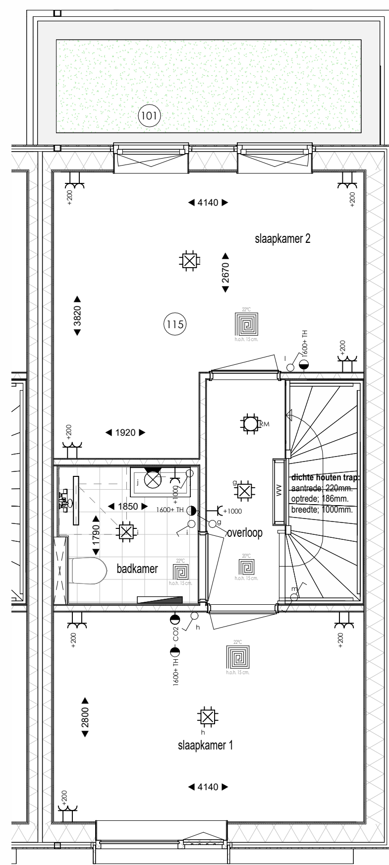
Eerste verdieping optie uitbouw 1.8m + slaapkamer samenvoegen
