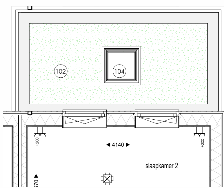
Eerste verdieping optie uitbouw 2.4m
