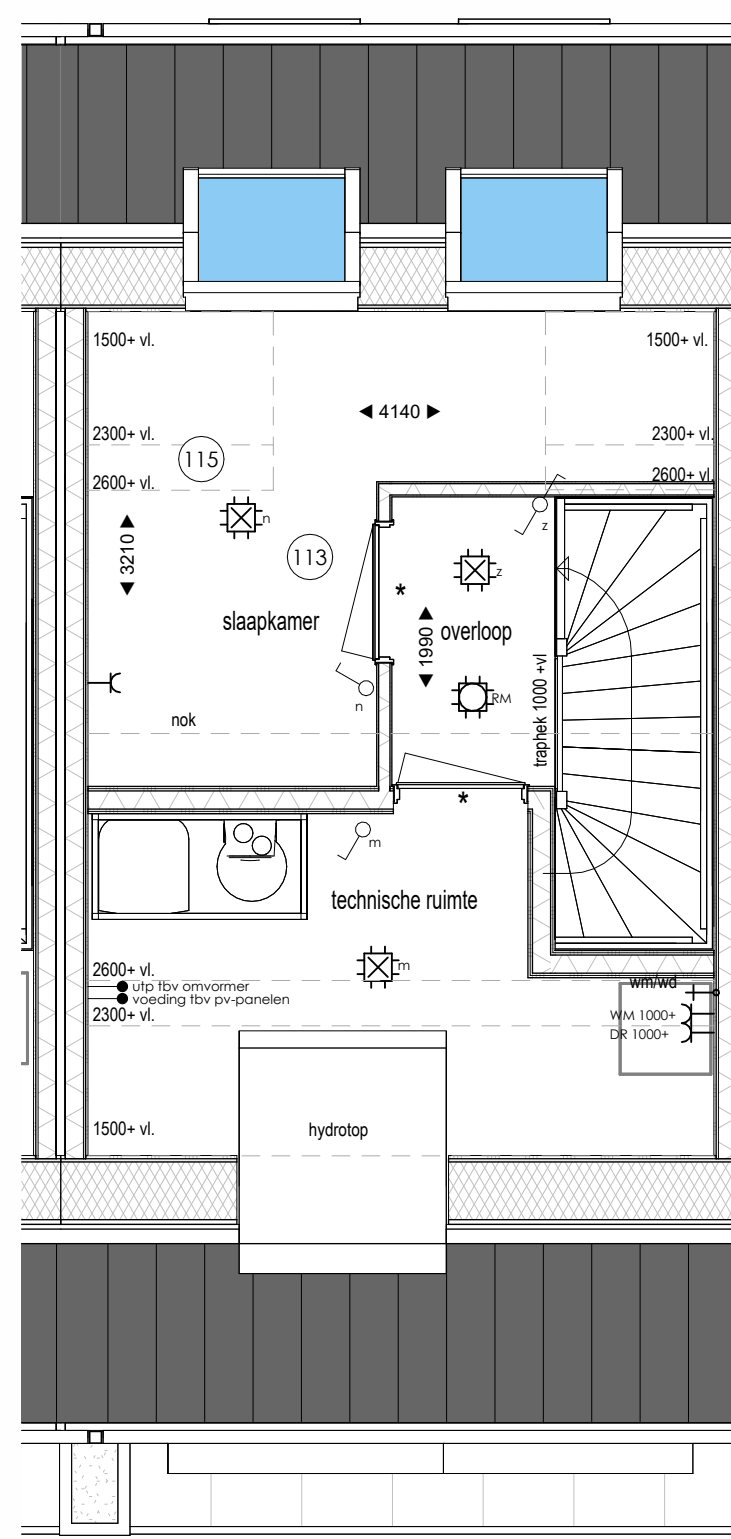
Tweede verdieping optie slaapkamer zolder met dakramen
