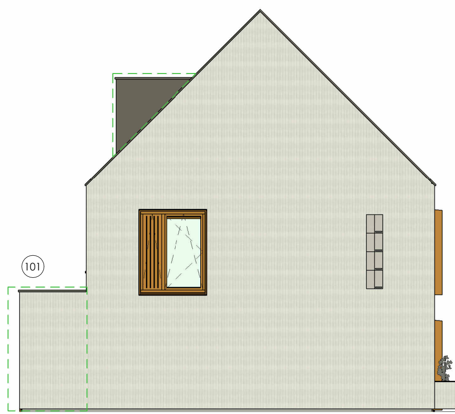
Linker zijgevel optie uitbouw 1,8m
