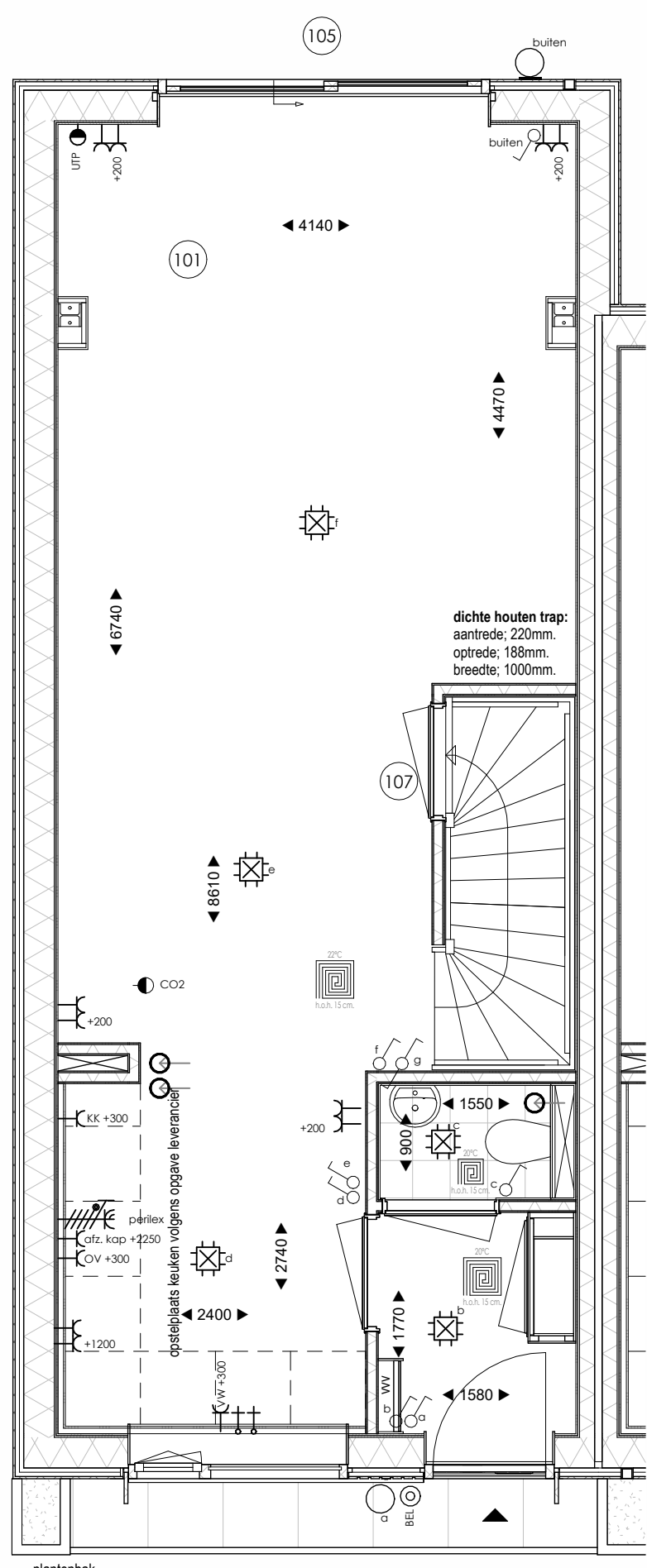
Begane grond optie uitbouw 1,8m + trapkast
