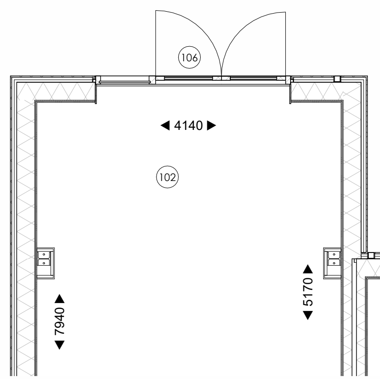
Begane grond optie uitbouw 2,4m
