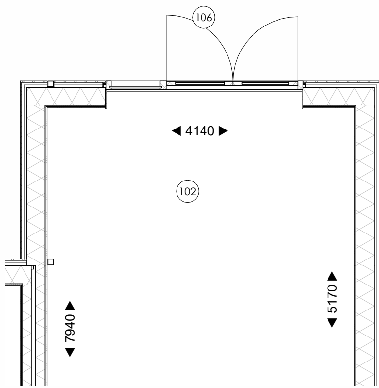
Begane grond optie uitbouw 2.4m
