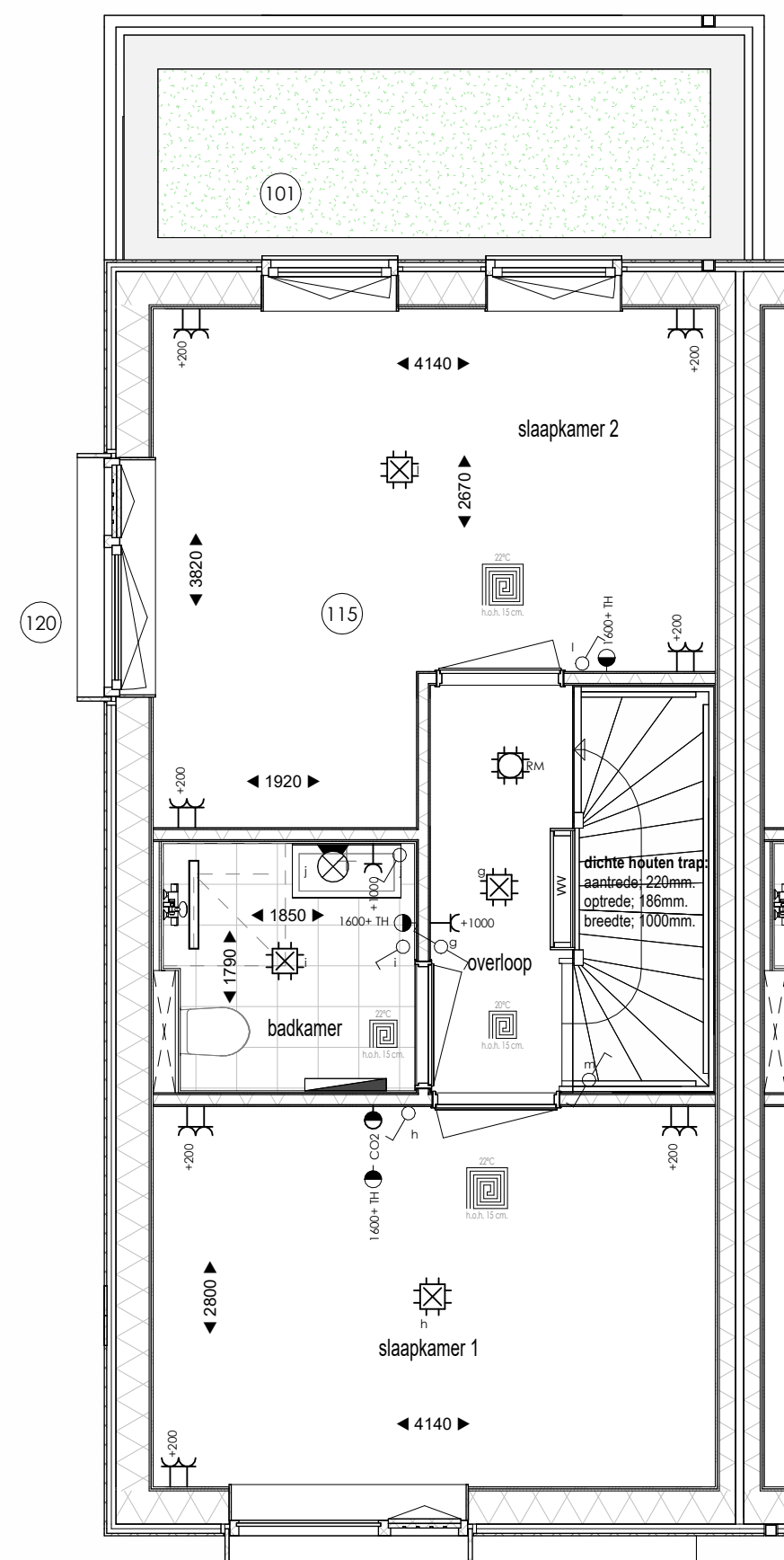
Eerste verdieping optie uitbouw 1,8m + slaapkamer samenvoegen
