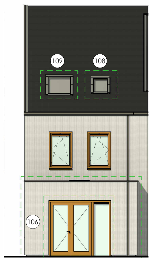
Achtergevel optie uitbouw 1.8m / 2.4m + dakramen + tuindeuren
