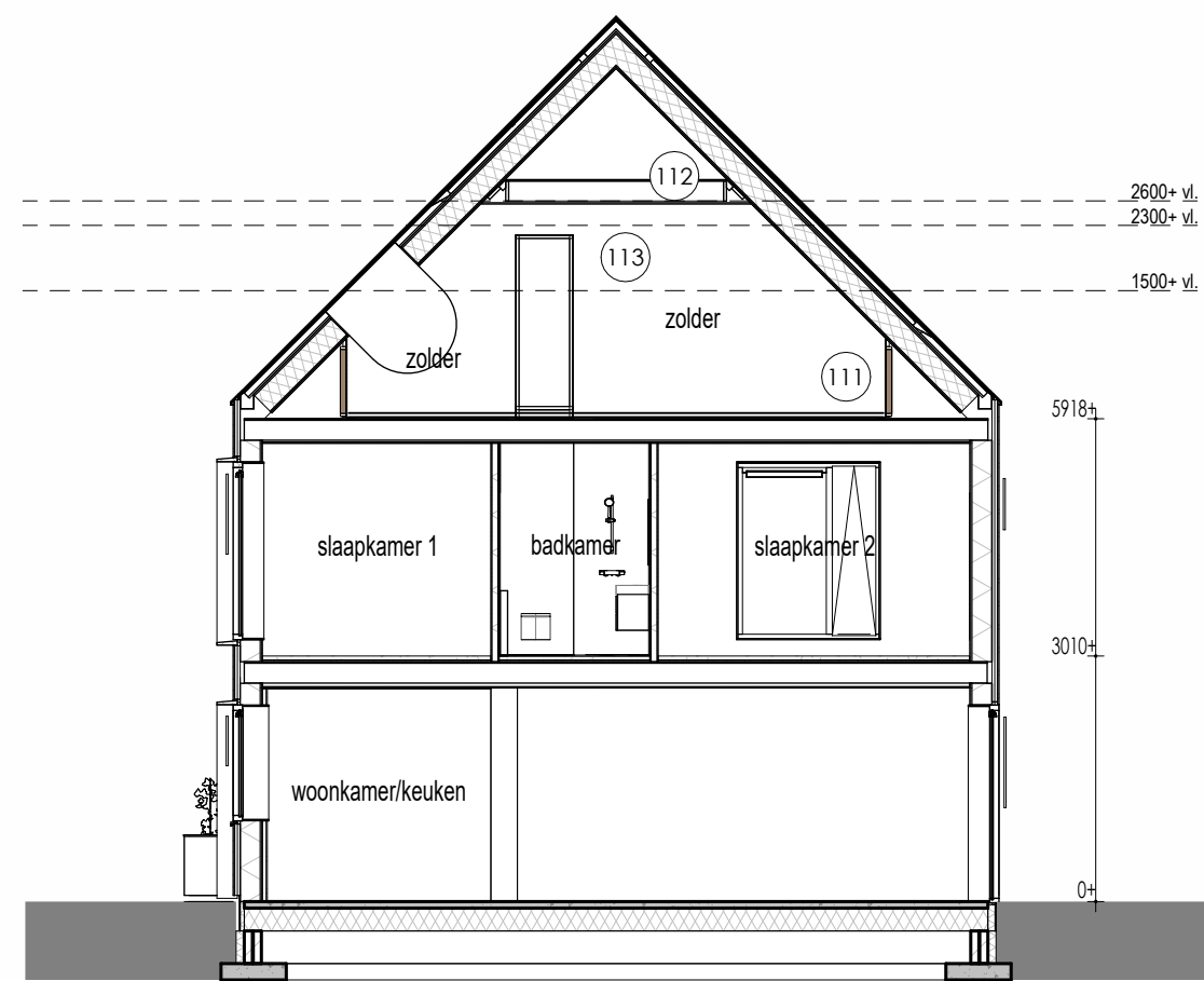
Doorsnede slaapkamer zolder + afwerking
