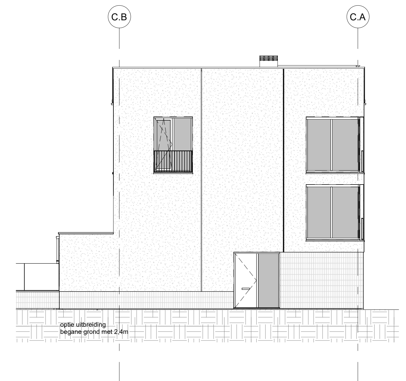
linker zijgevel blok 12c (Noord-West) opties
