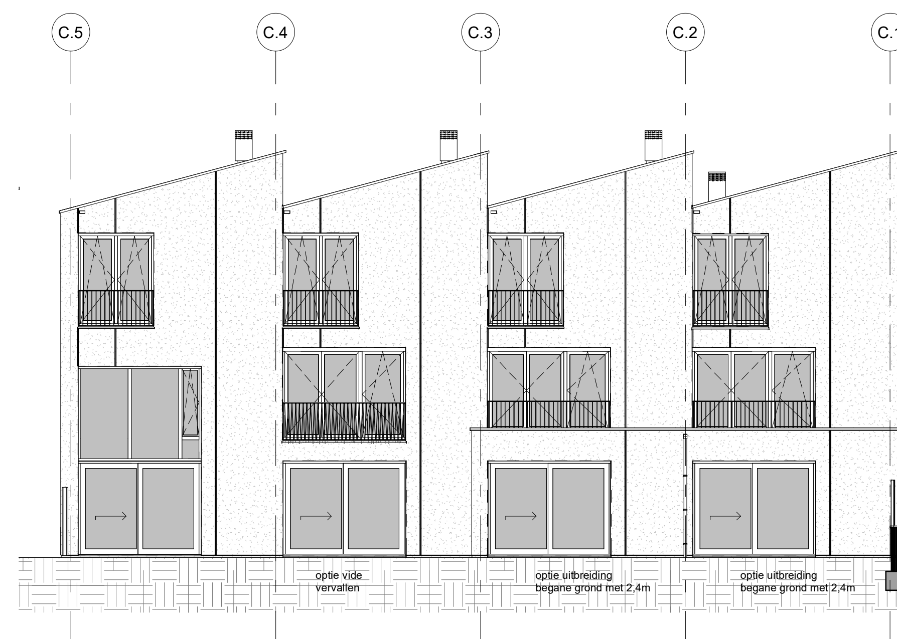
Achtergevel blok 12c (Noord-Oost) opties
