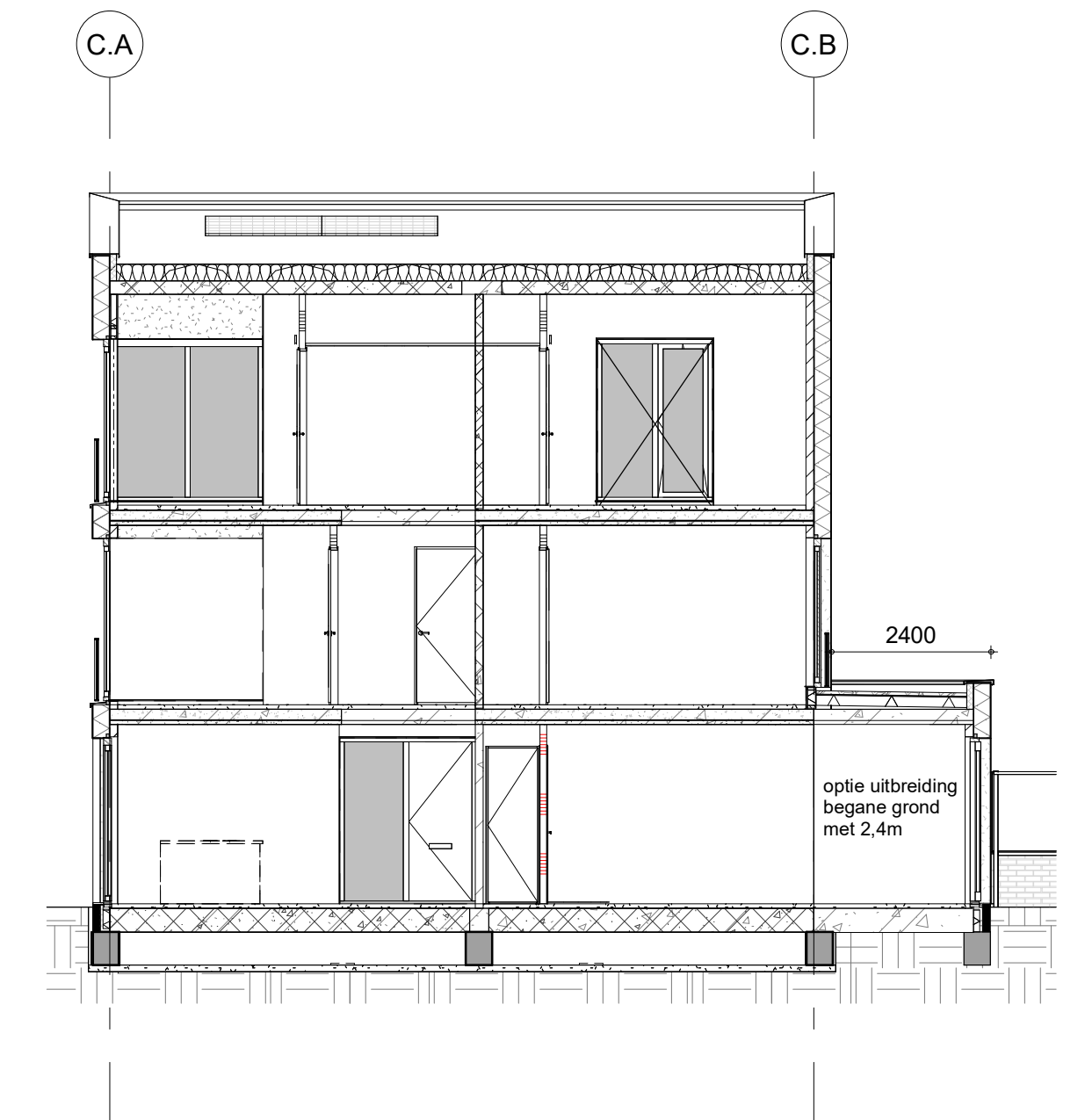
Doorsnede 12c.bo
