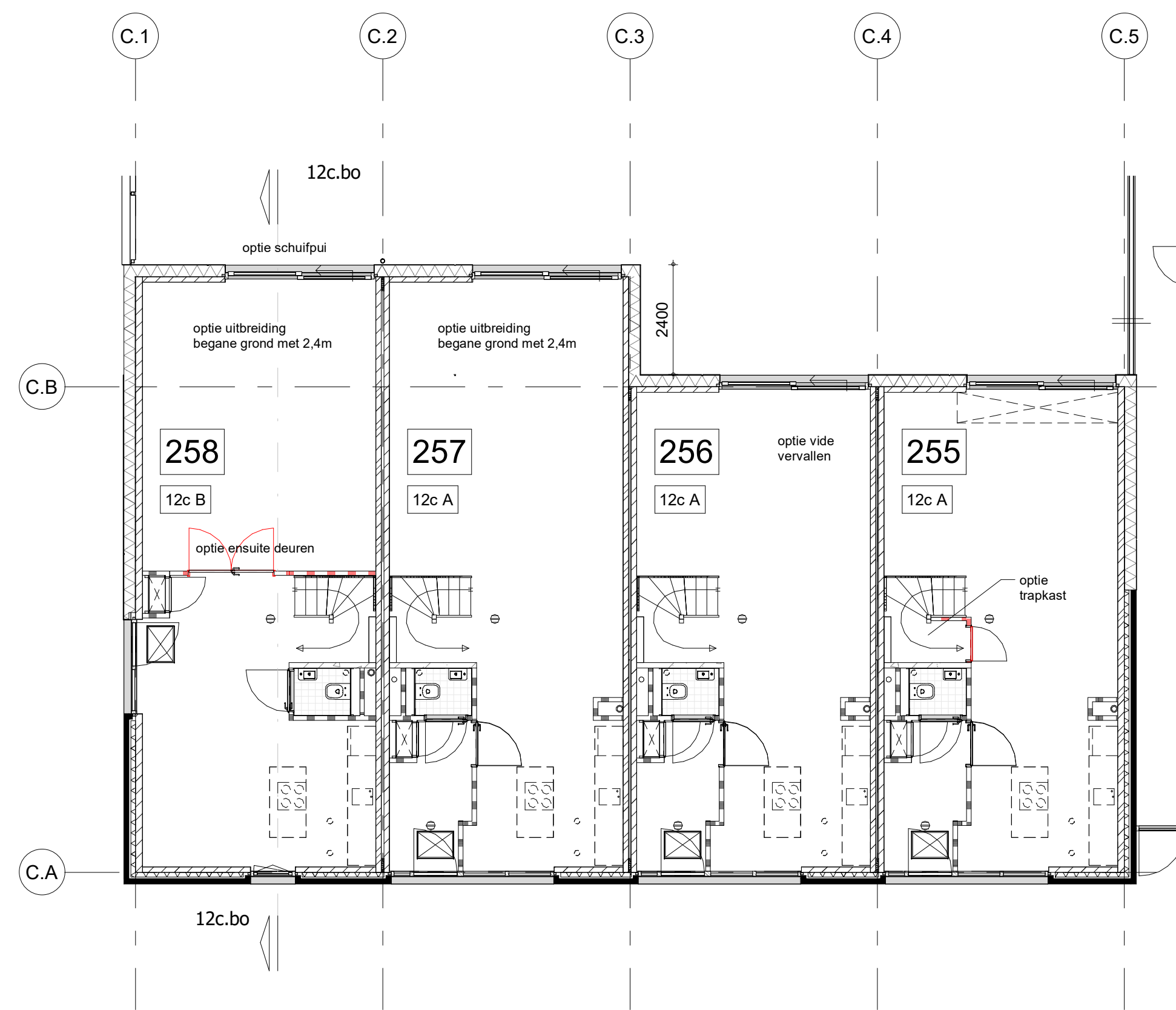
begane grond blok 12c opties
