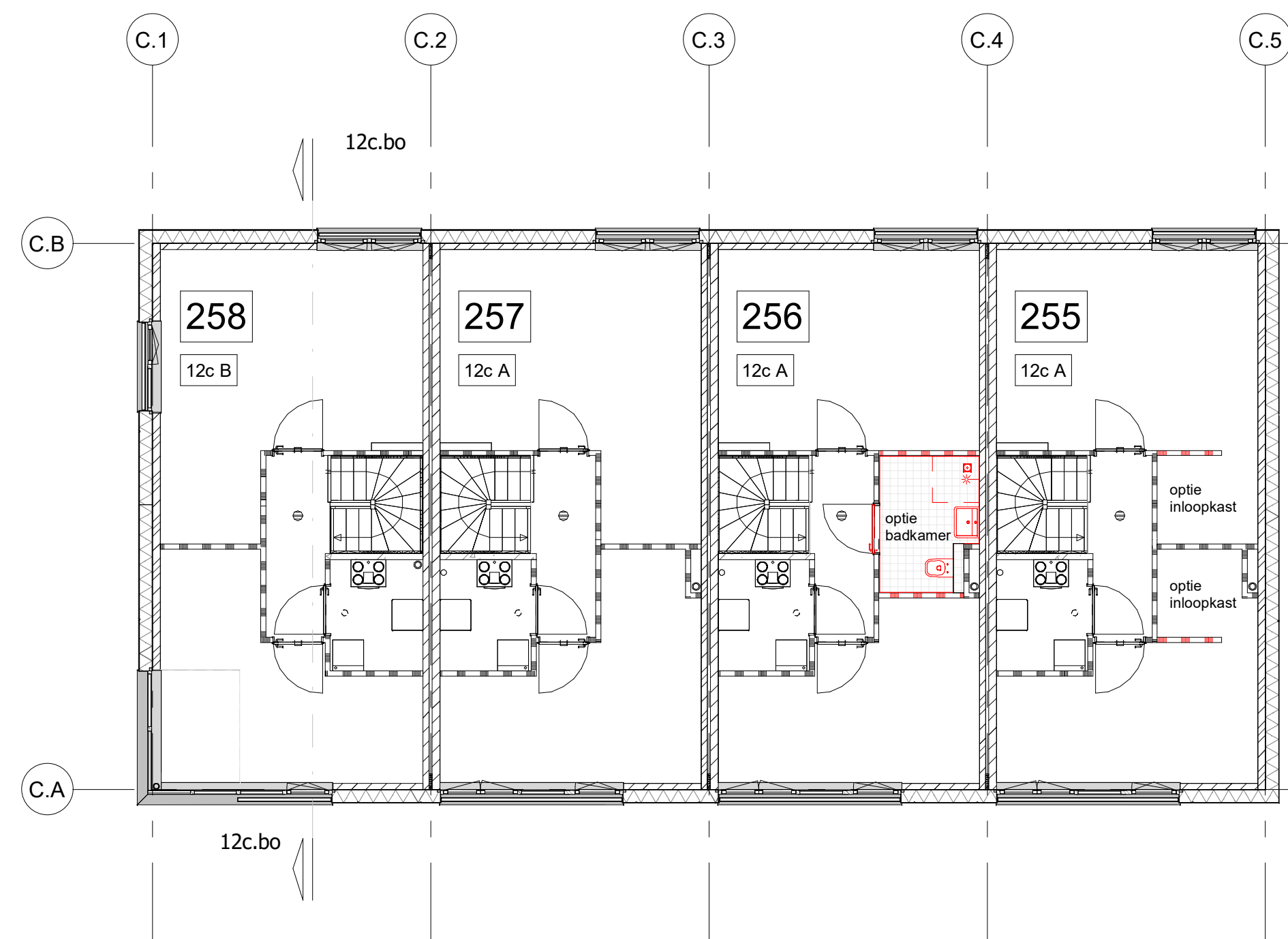
tweede verdieping blok 12c opties
