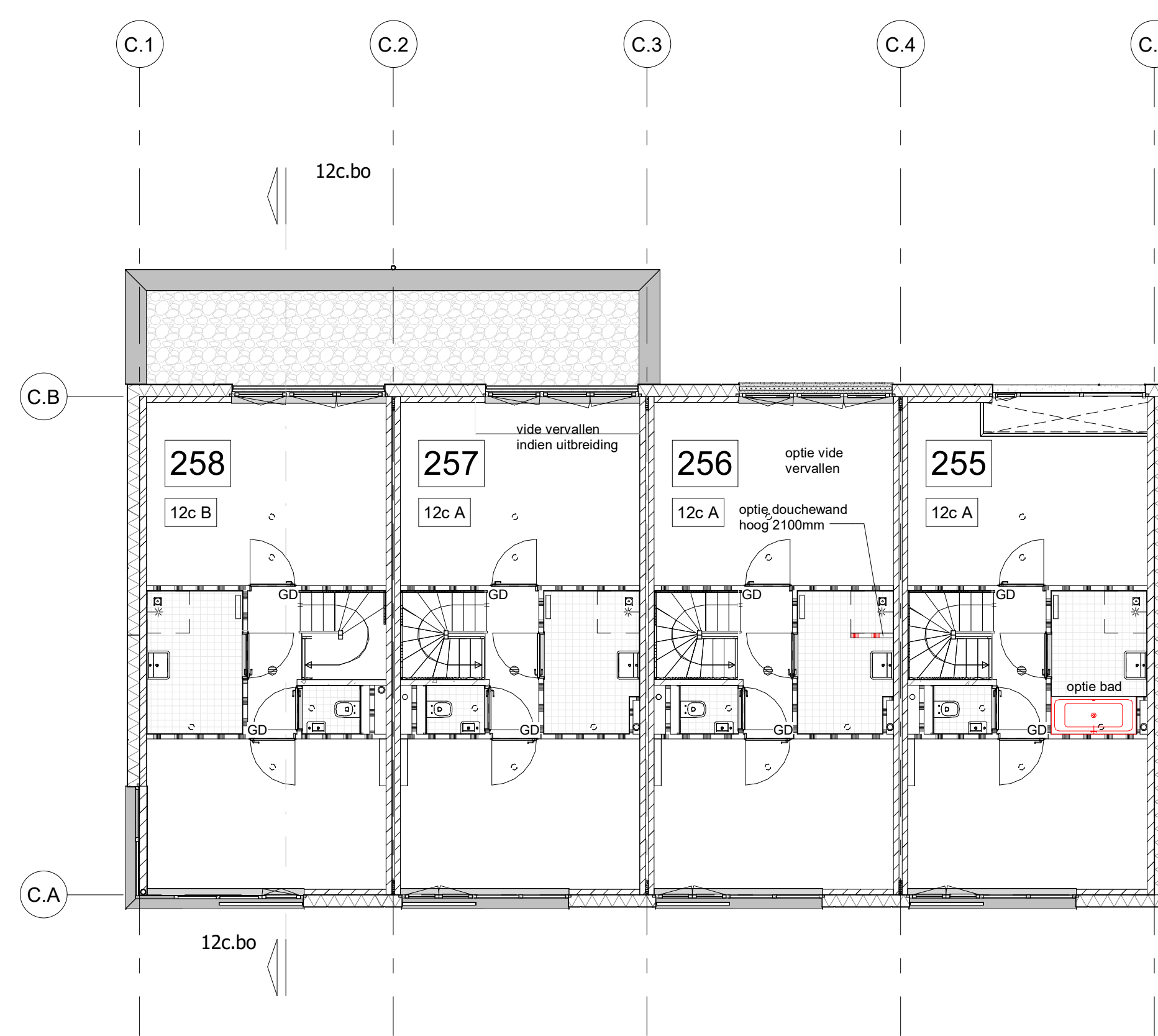
eerste verdieping blok 12c opties
