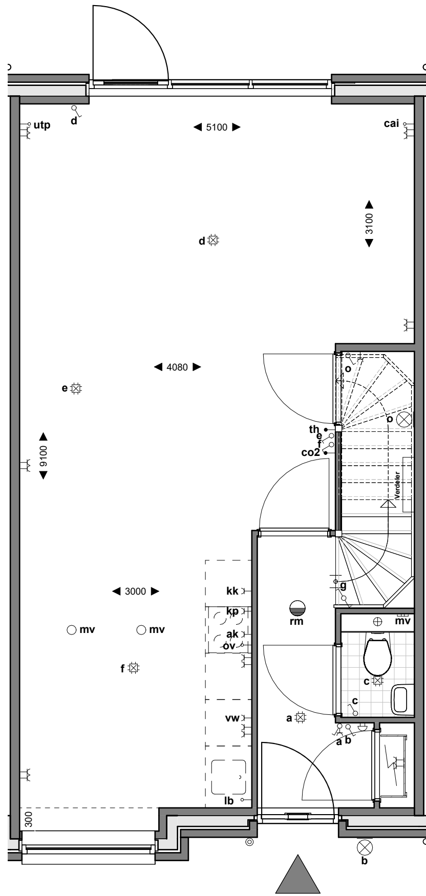
begane grond
