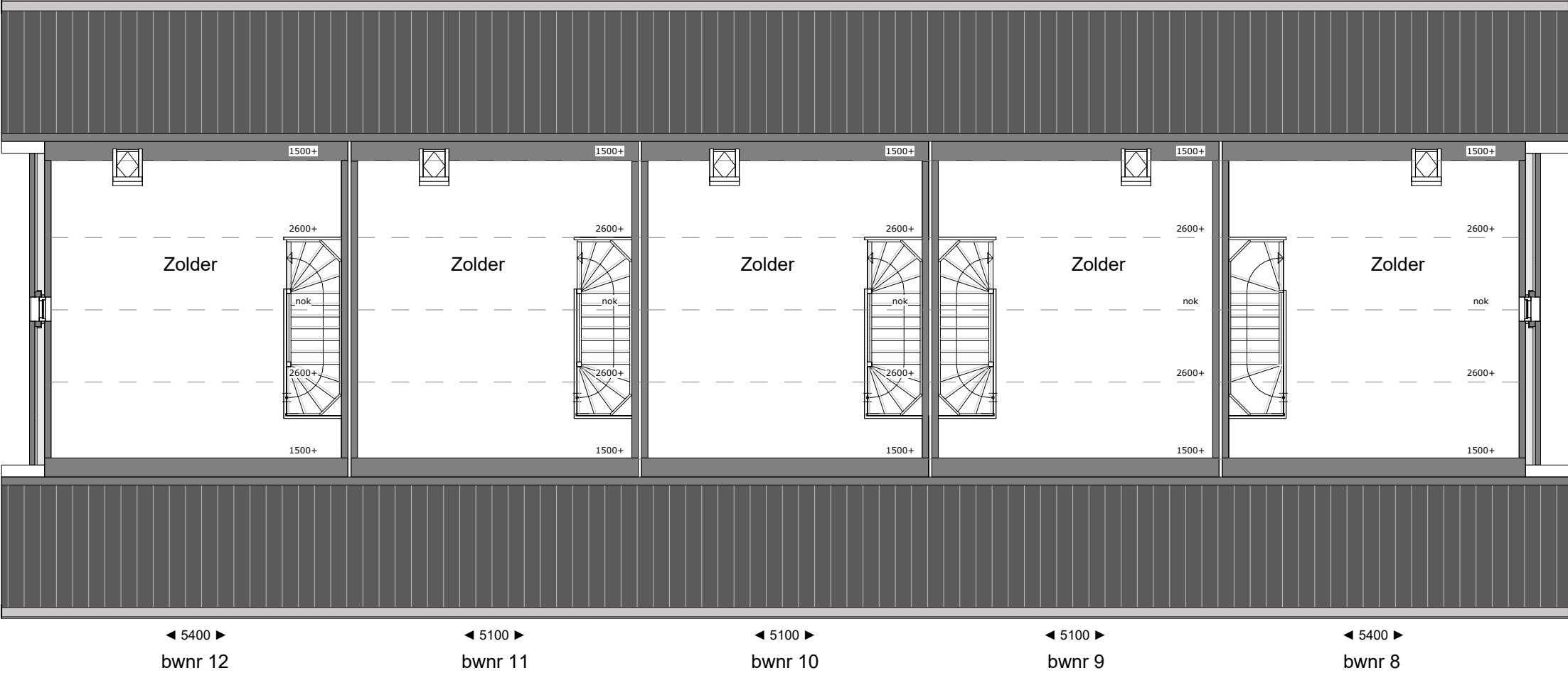
tweede verdieping
