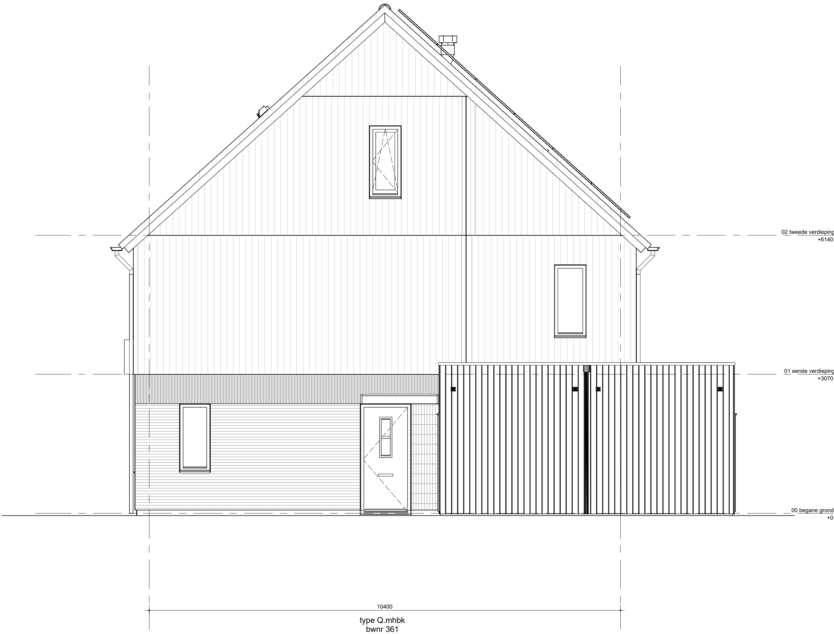
zijgevel rechts blok 10.3
