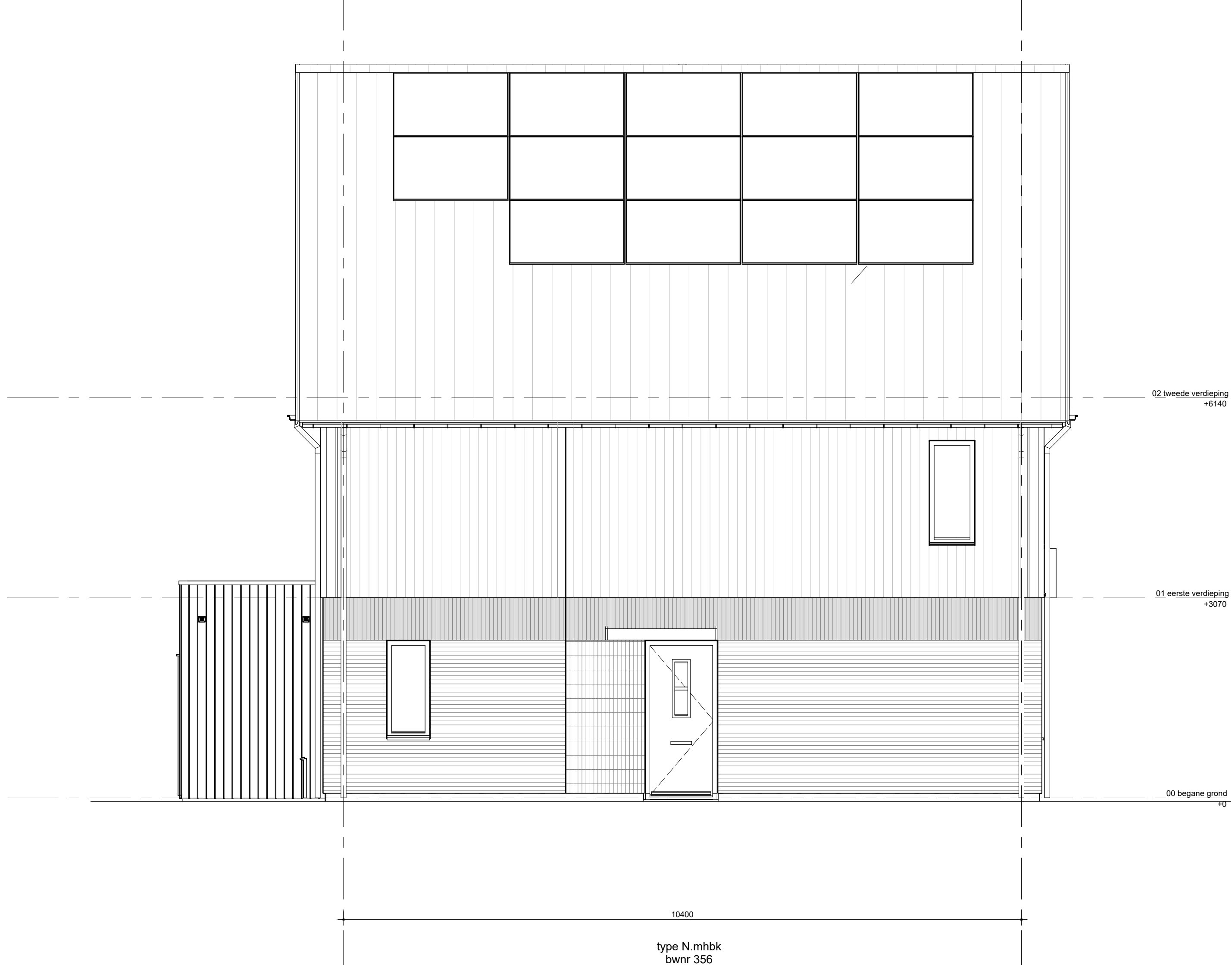
zijgevel links blok 10.1
