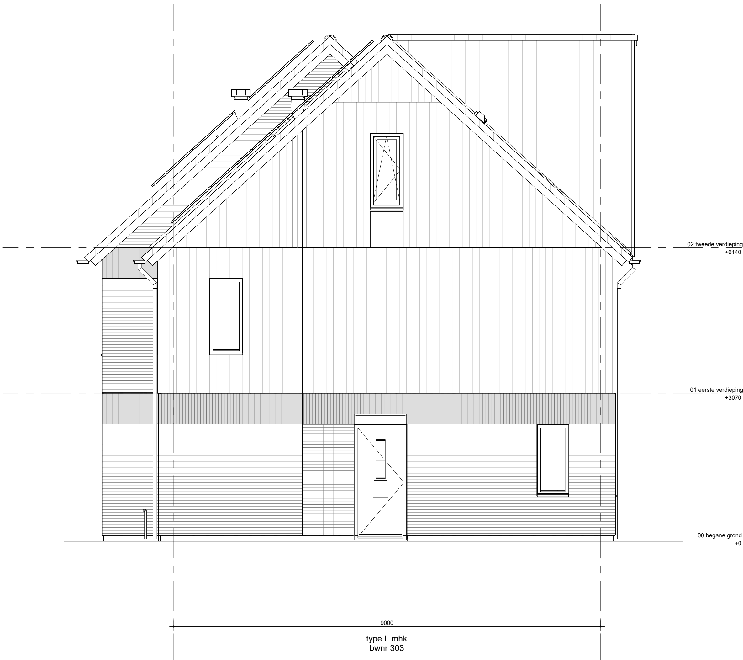
zijgevel links blok 02
