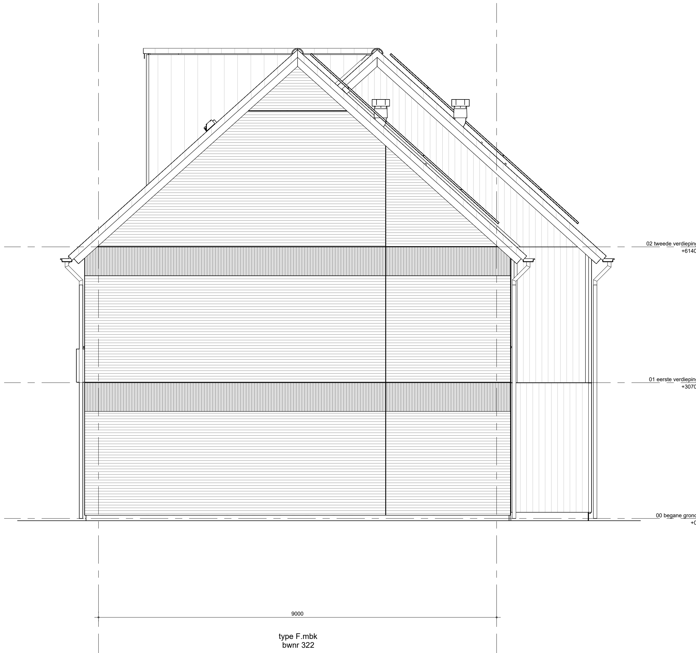
zijaanzicht rechts blok 04
