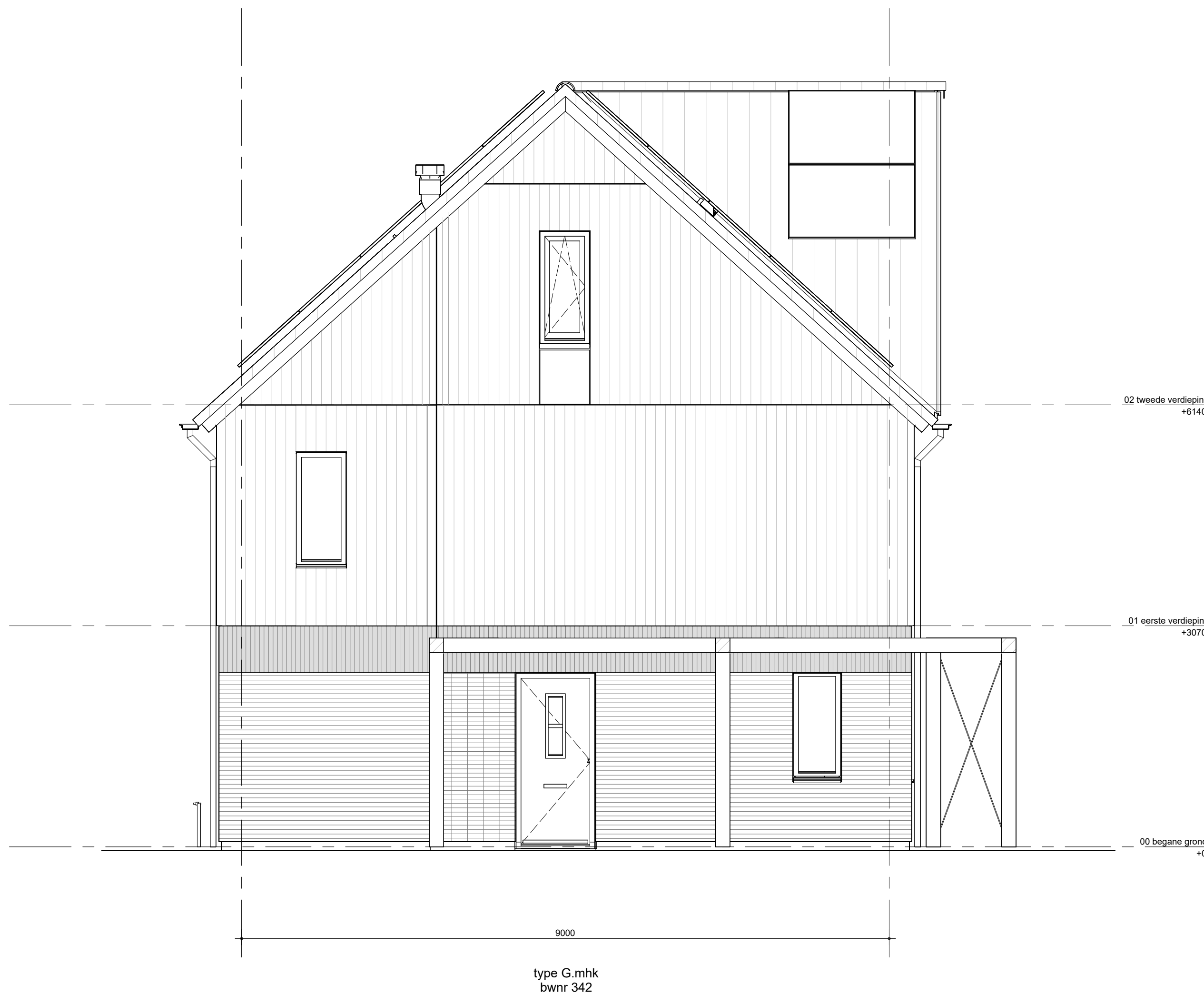
zijaanzicht rechts blok 08
