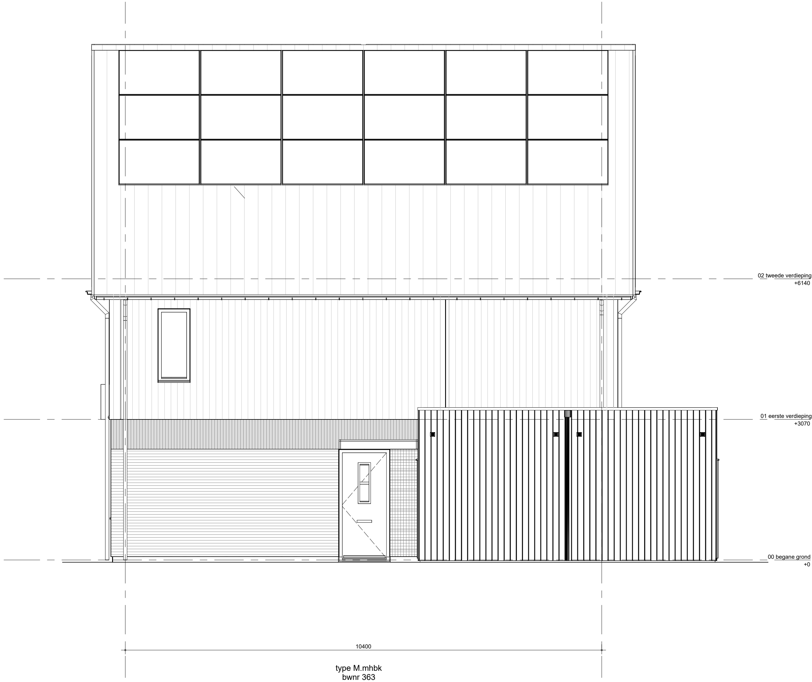
zijgevel rechts blok 10.4
