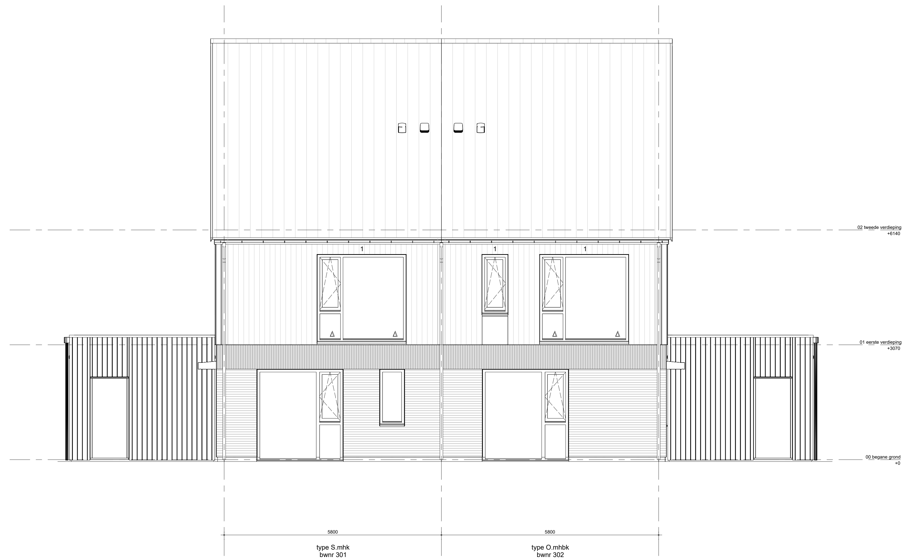
voorgevel blok 01
