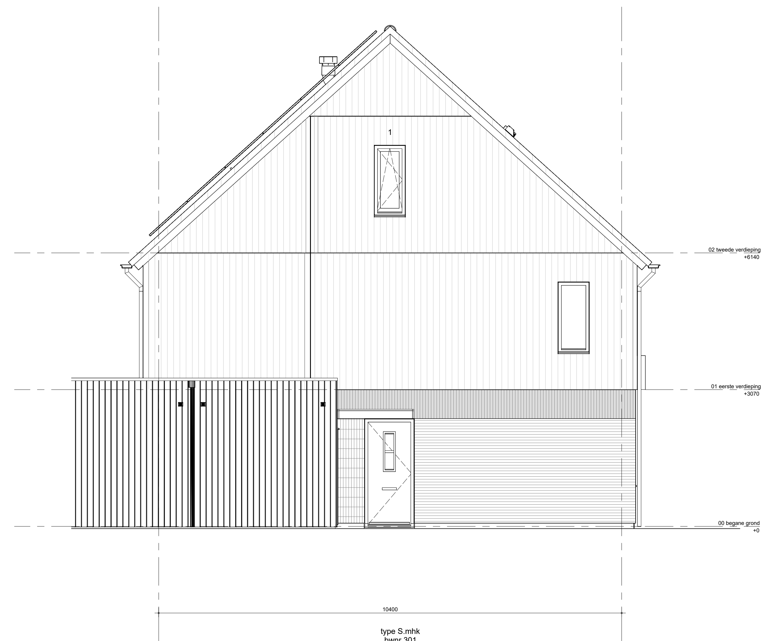
zijgevel links blok 01
