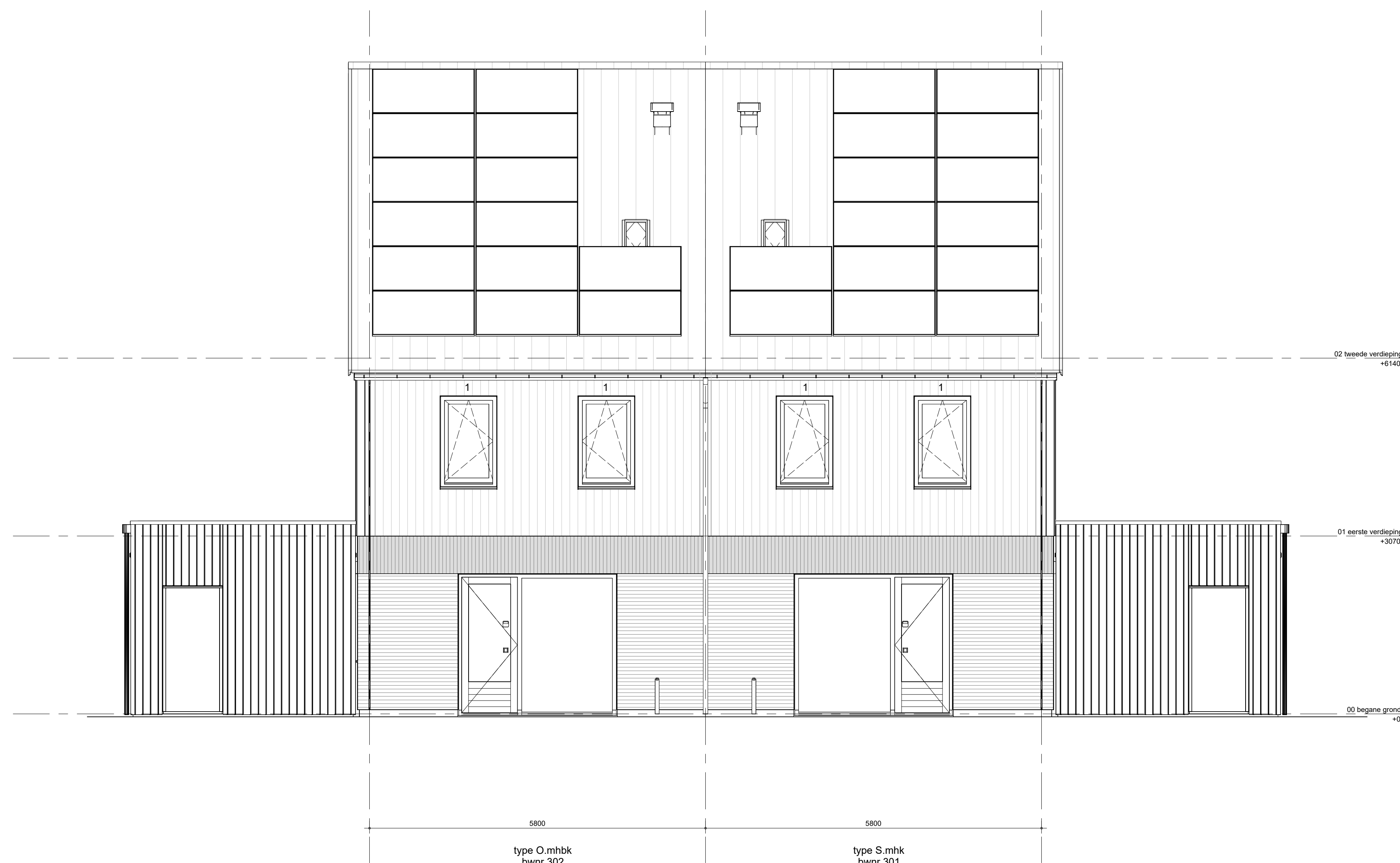
achtergevel blok 01
