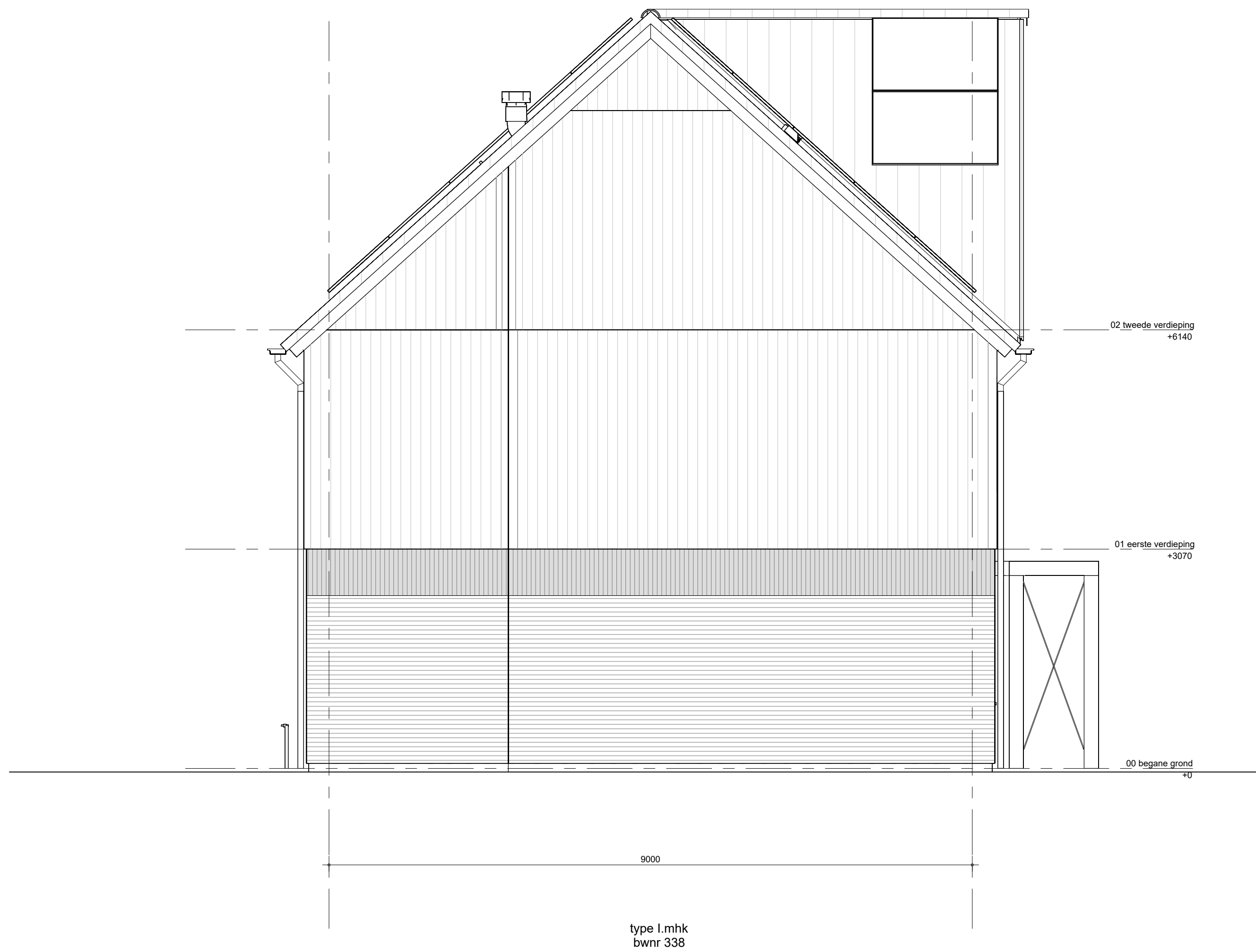
zijgevel links blok 07
