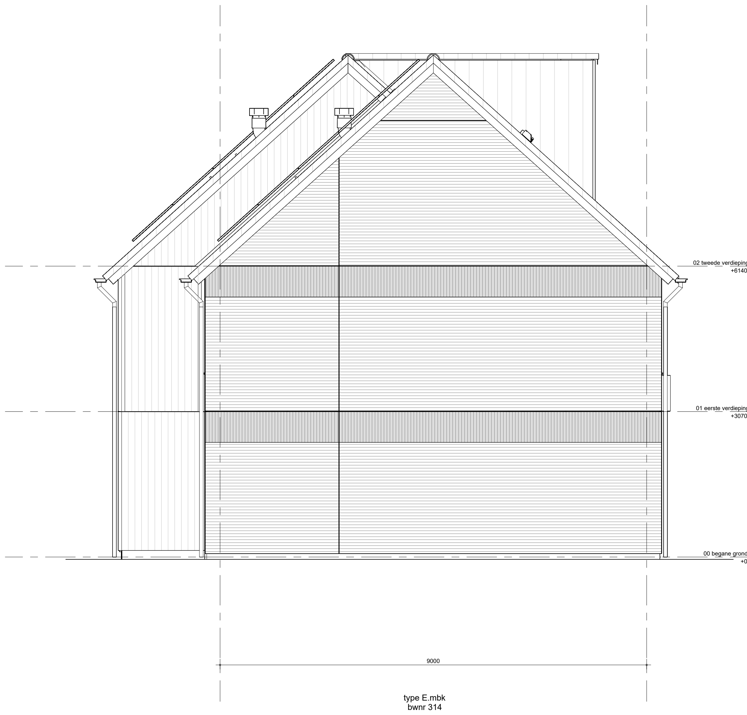
zijaanzicht links blok 04
