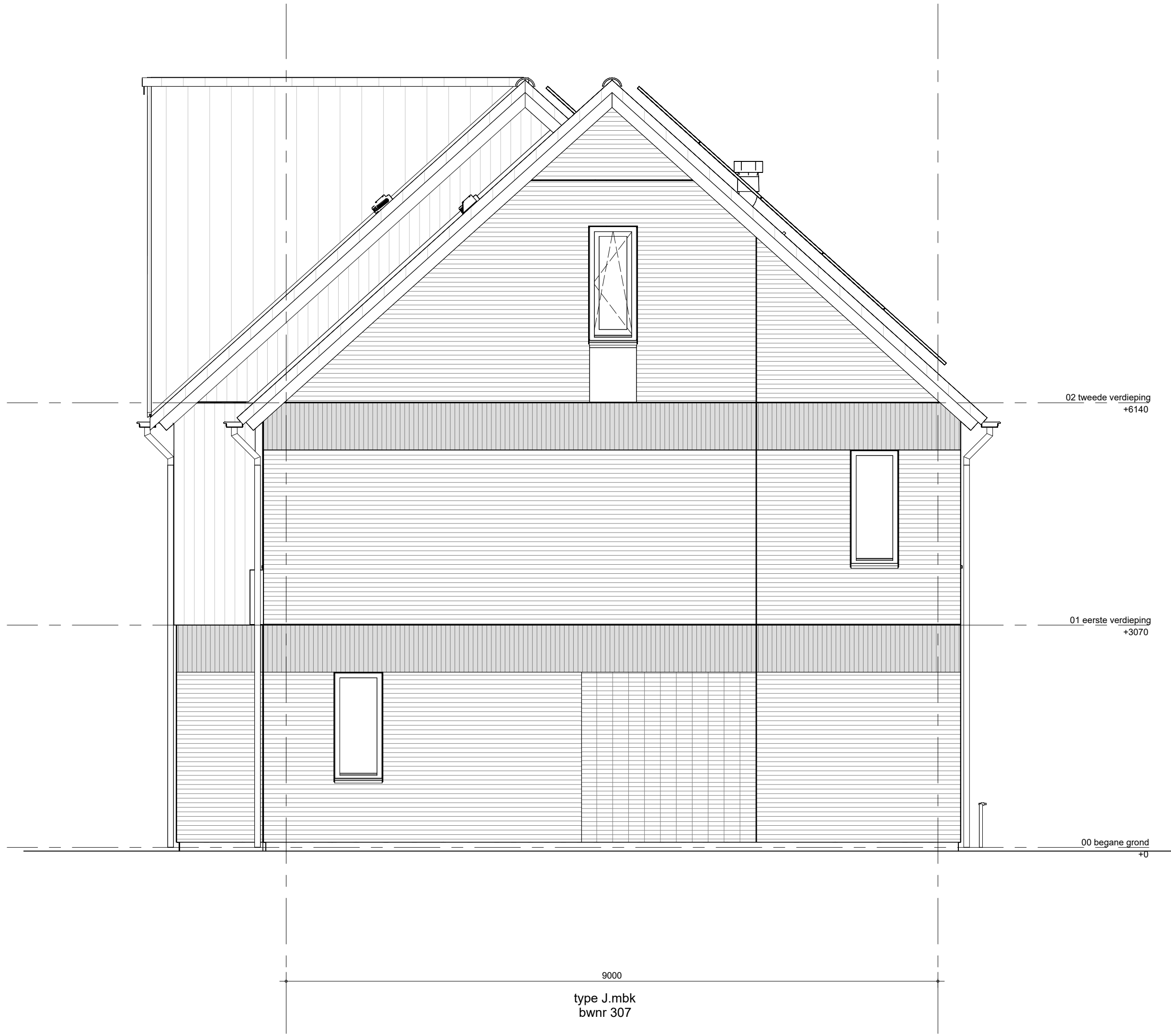
zijgevel rechts blok 02
