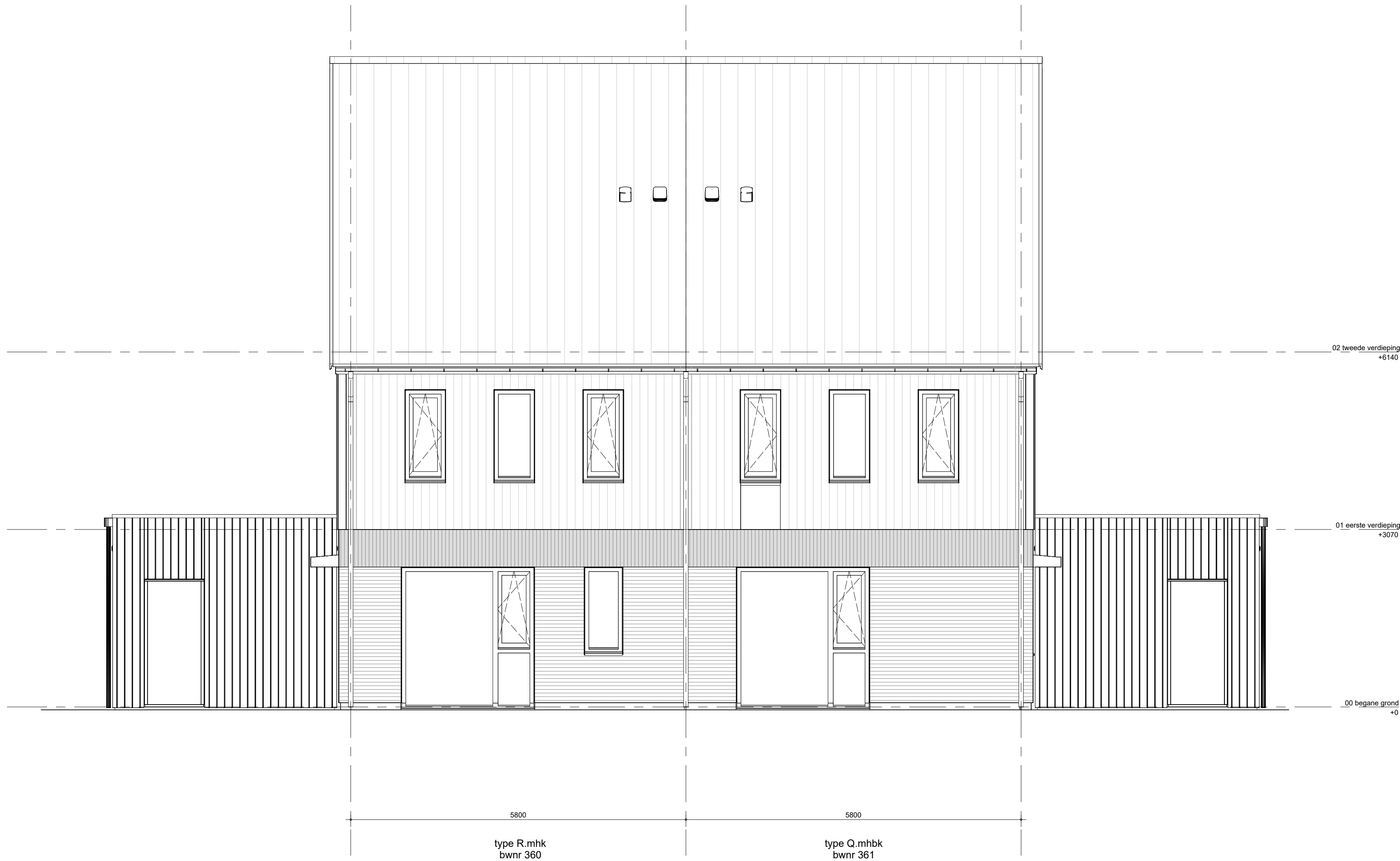
voorgevel blok 10.3
