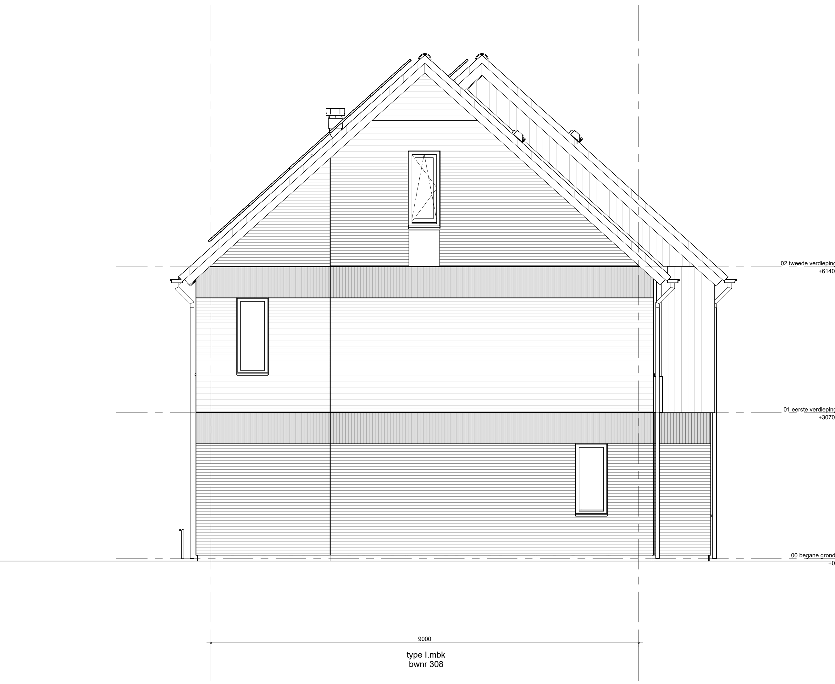
zijgevel links blok 03
