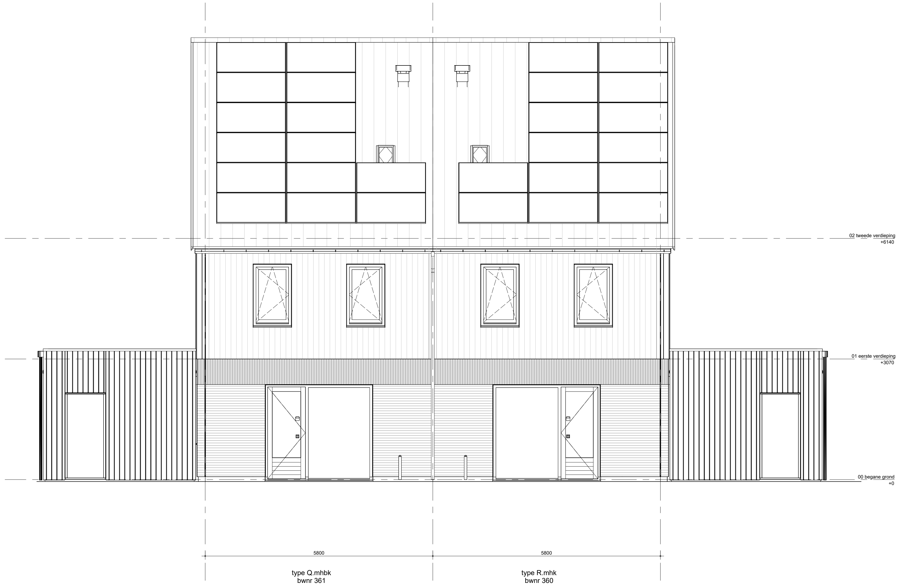
achtergevel blok 10.3
