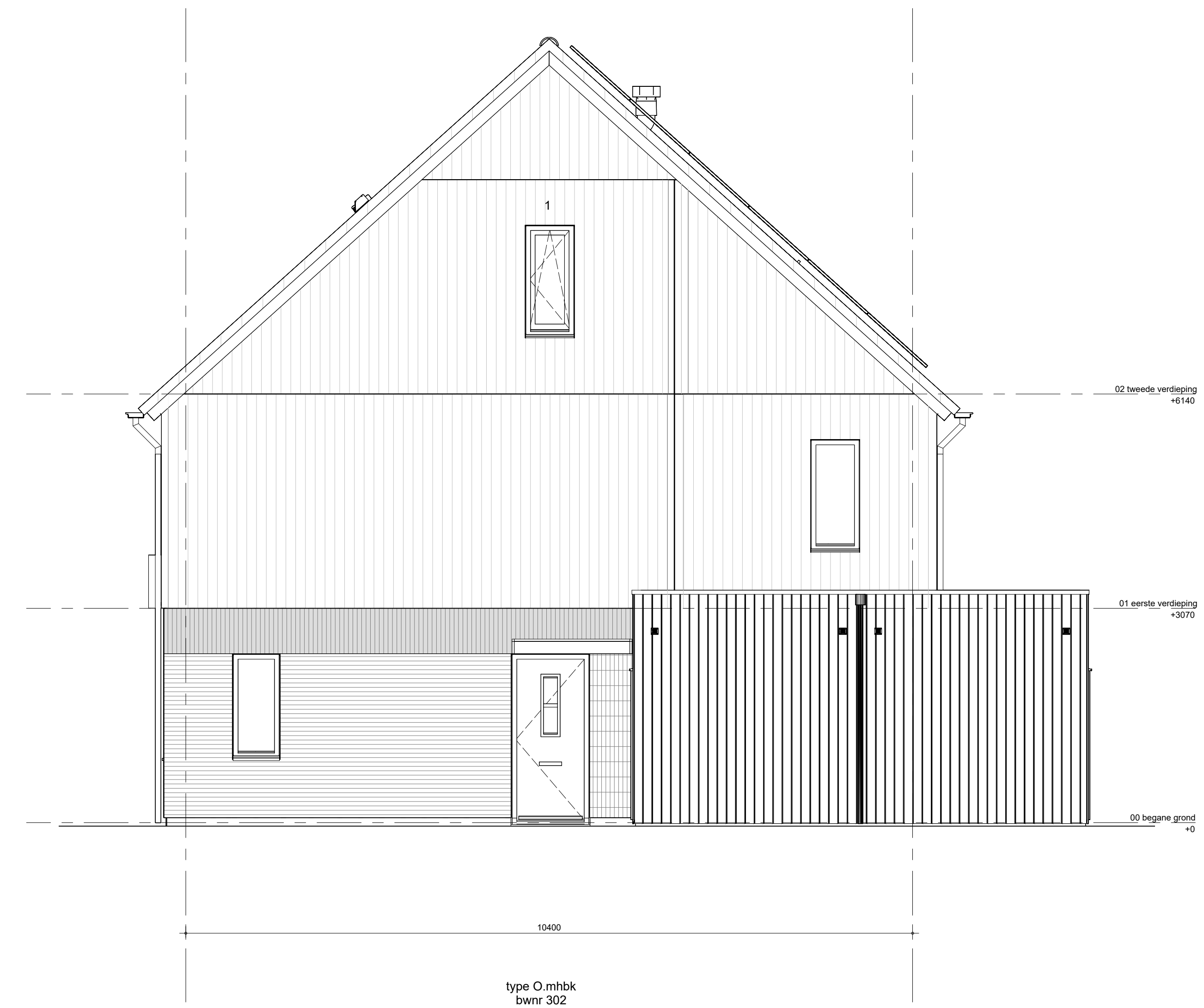
zijgevel rechts blok 01
