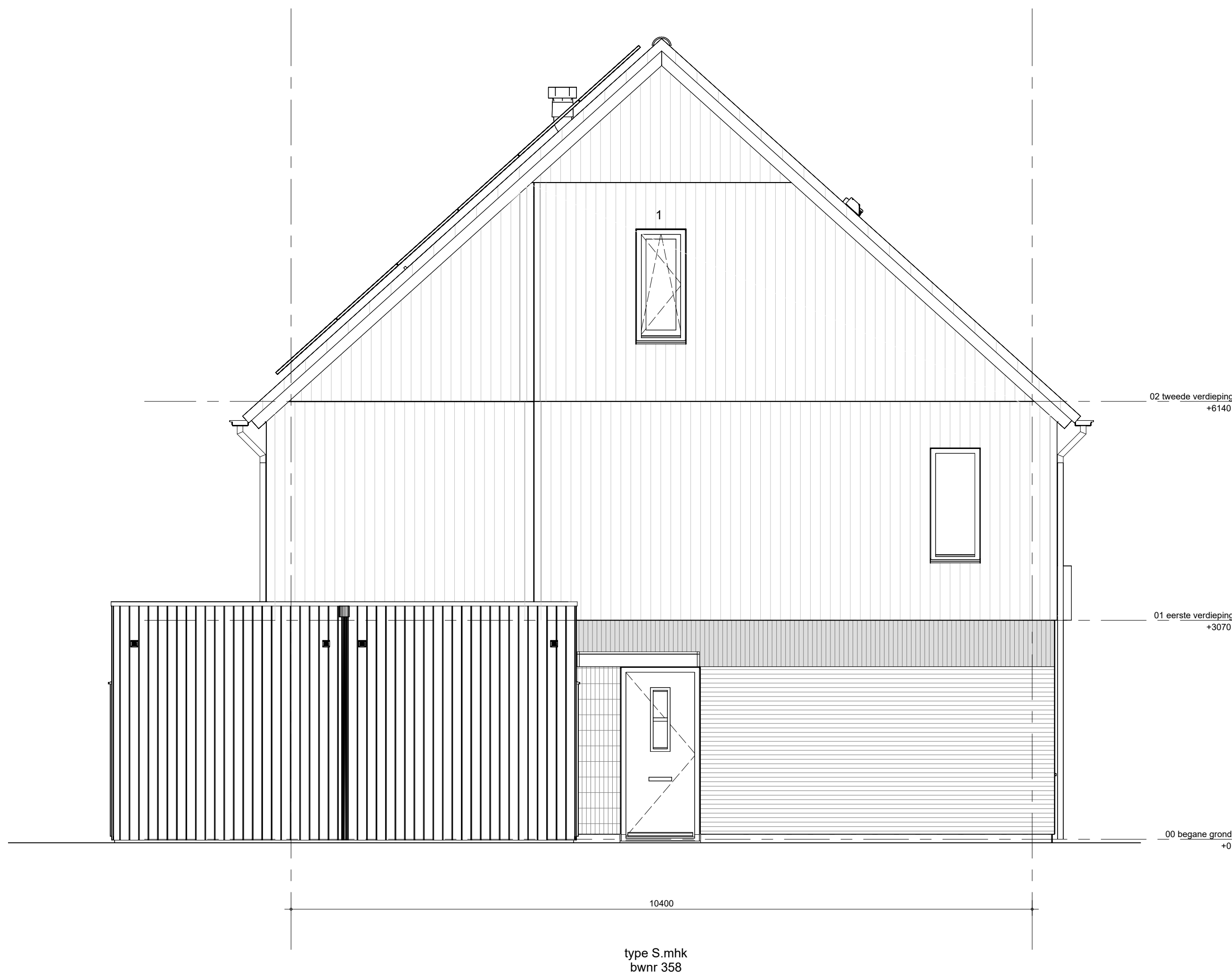
zijgevel links blok 10.2
