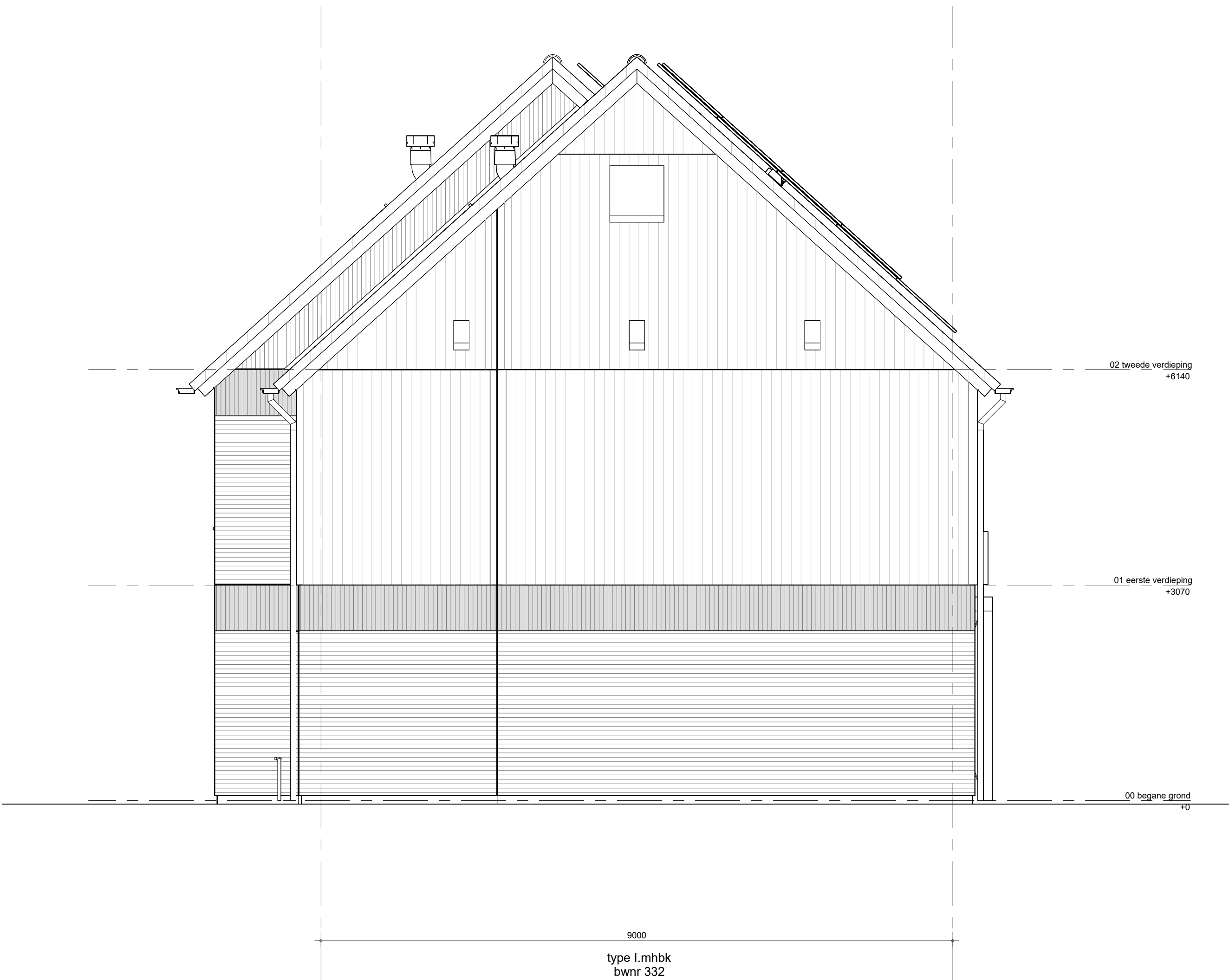
zijgevel links blok 06
