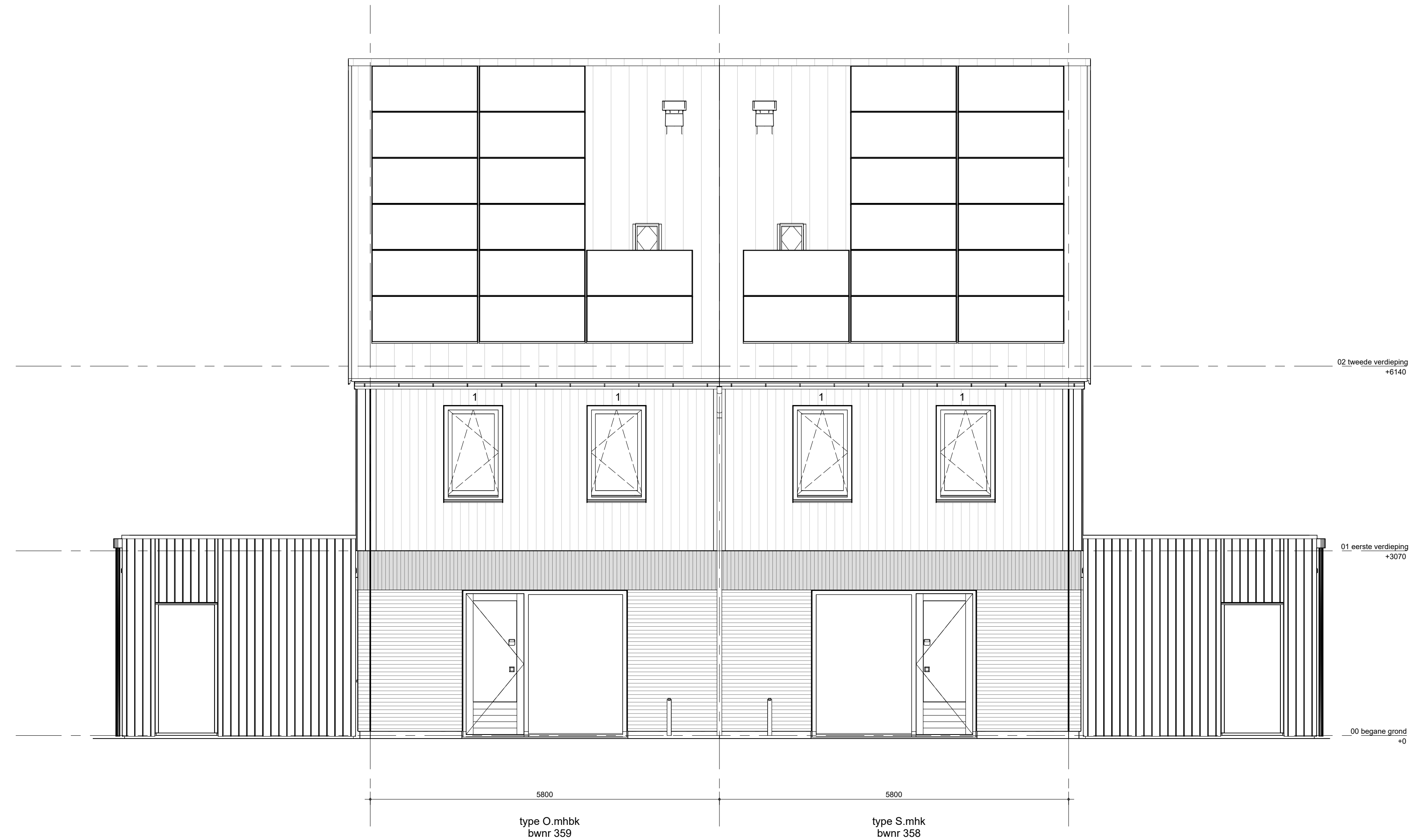
achtergevel blok 10.2
