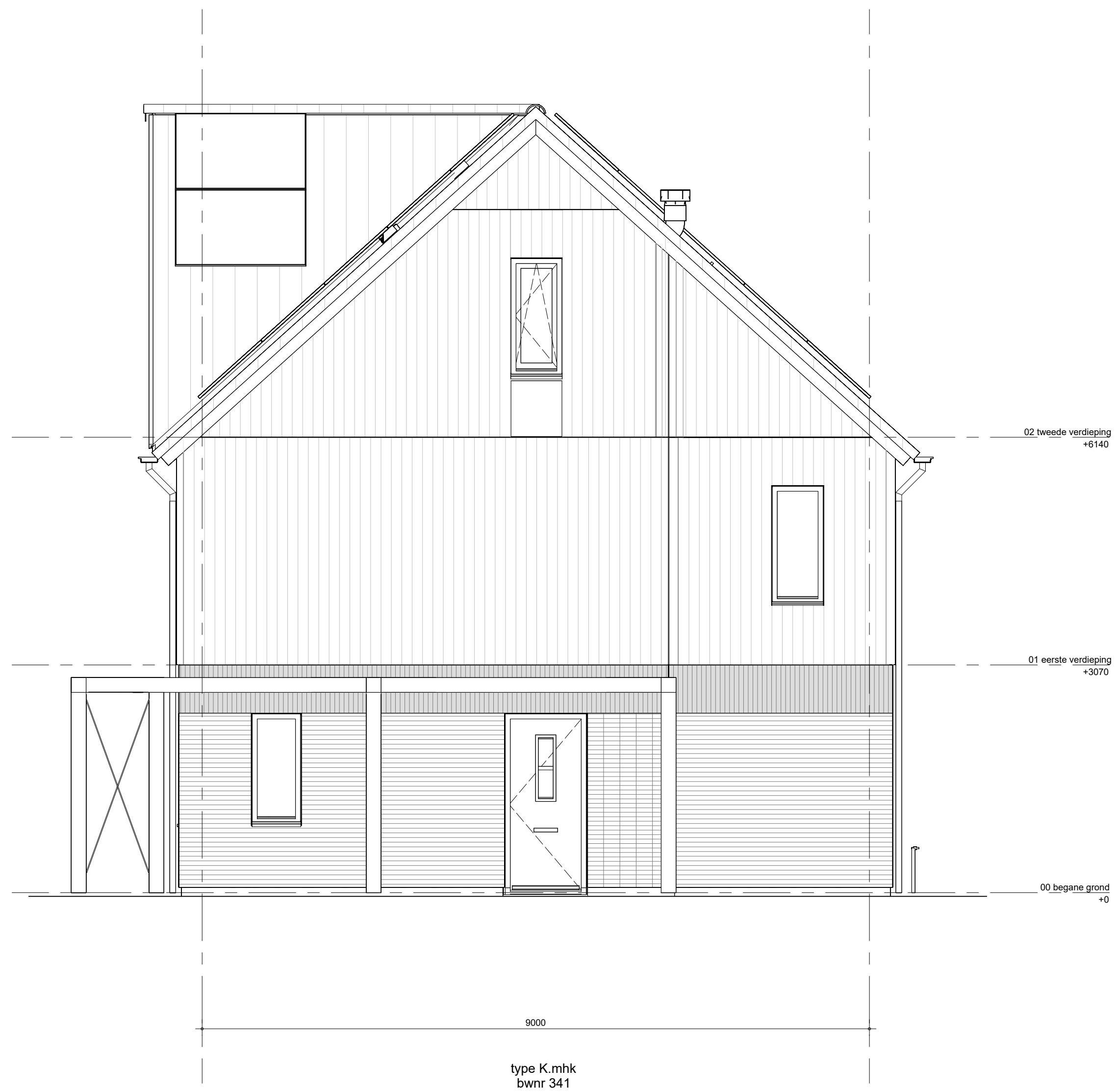
zijgevel rechts blok 07
