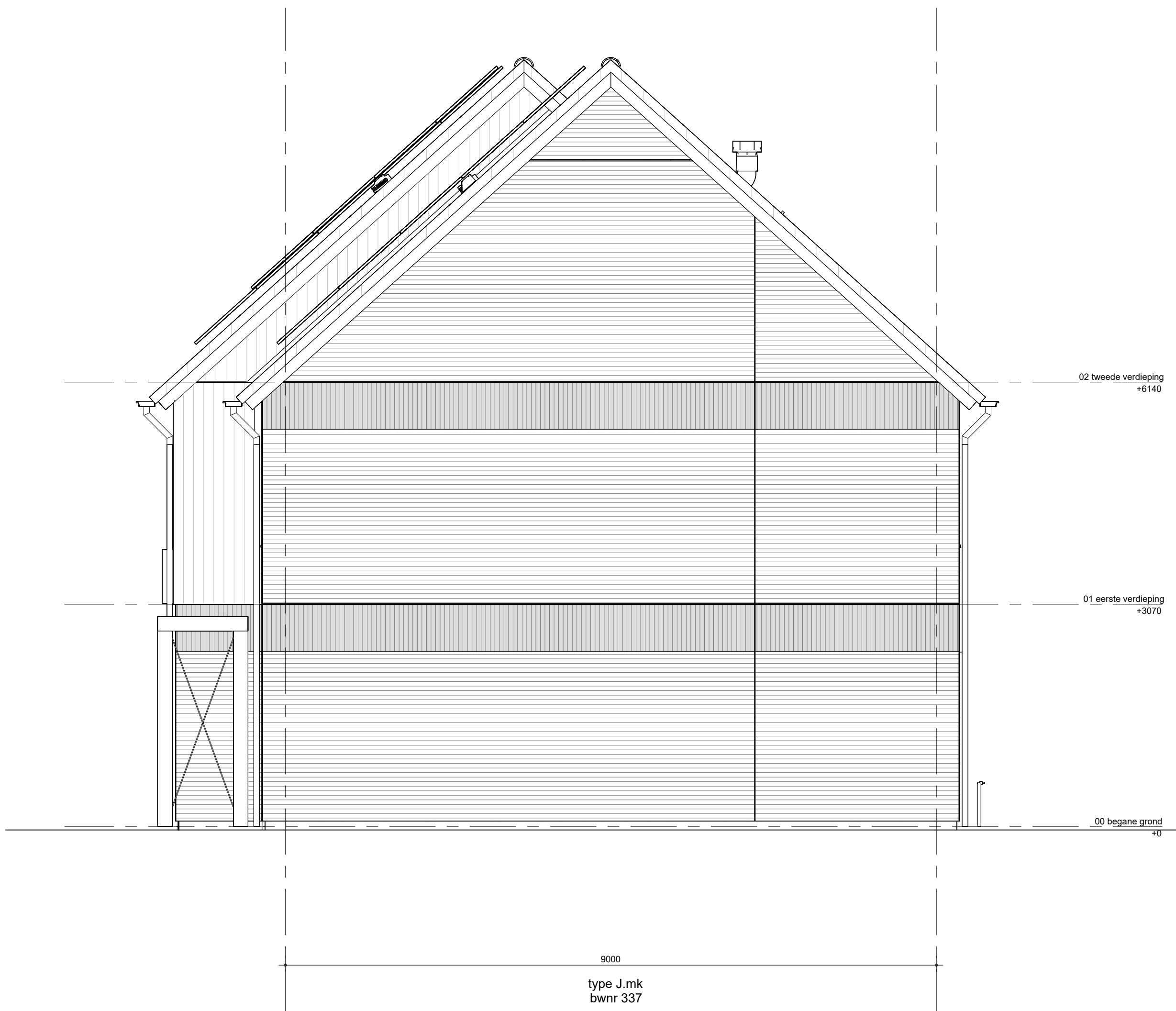
zijgevel rechts blok 06
