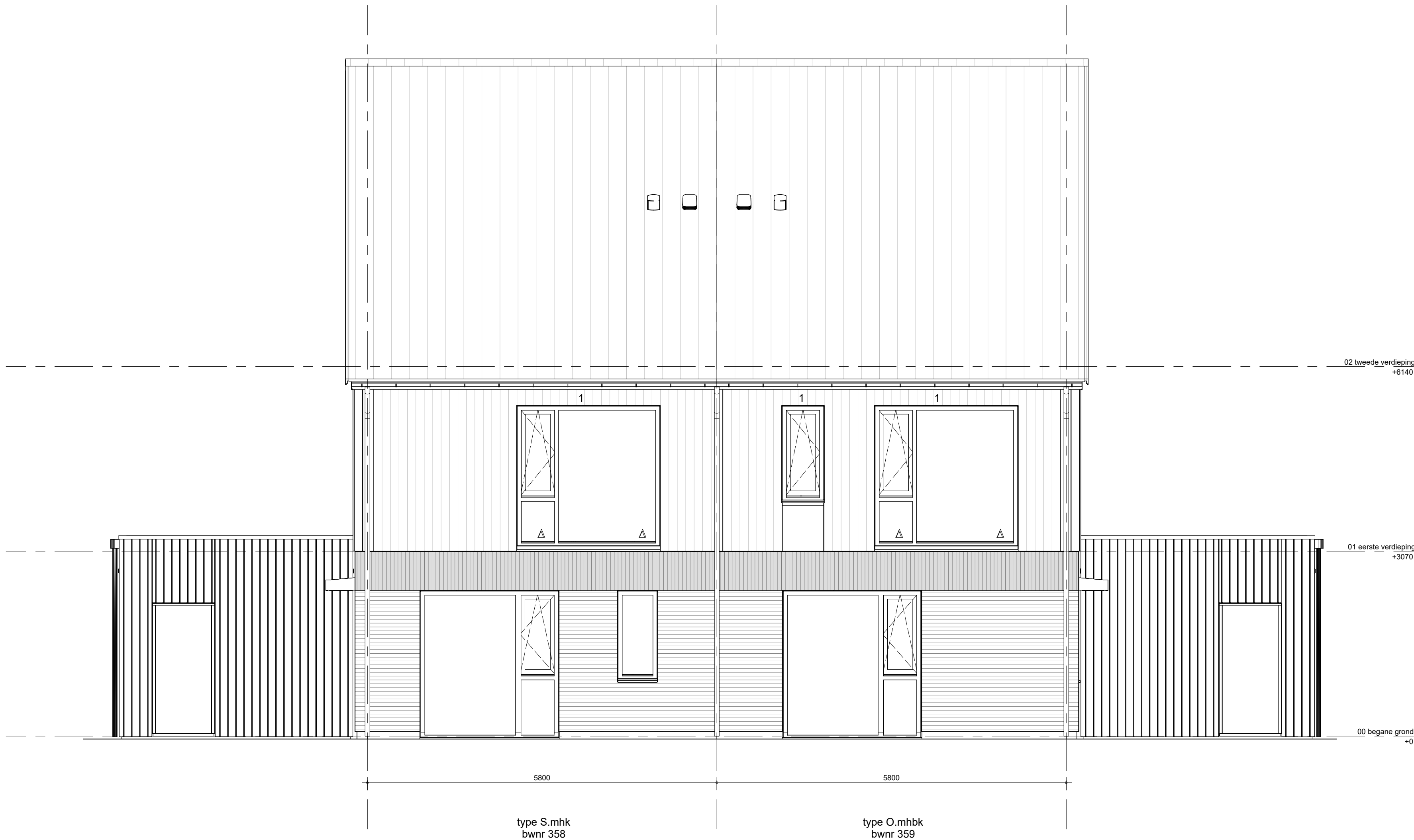
voorgevel blok 10.2
