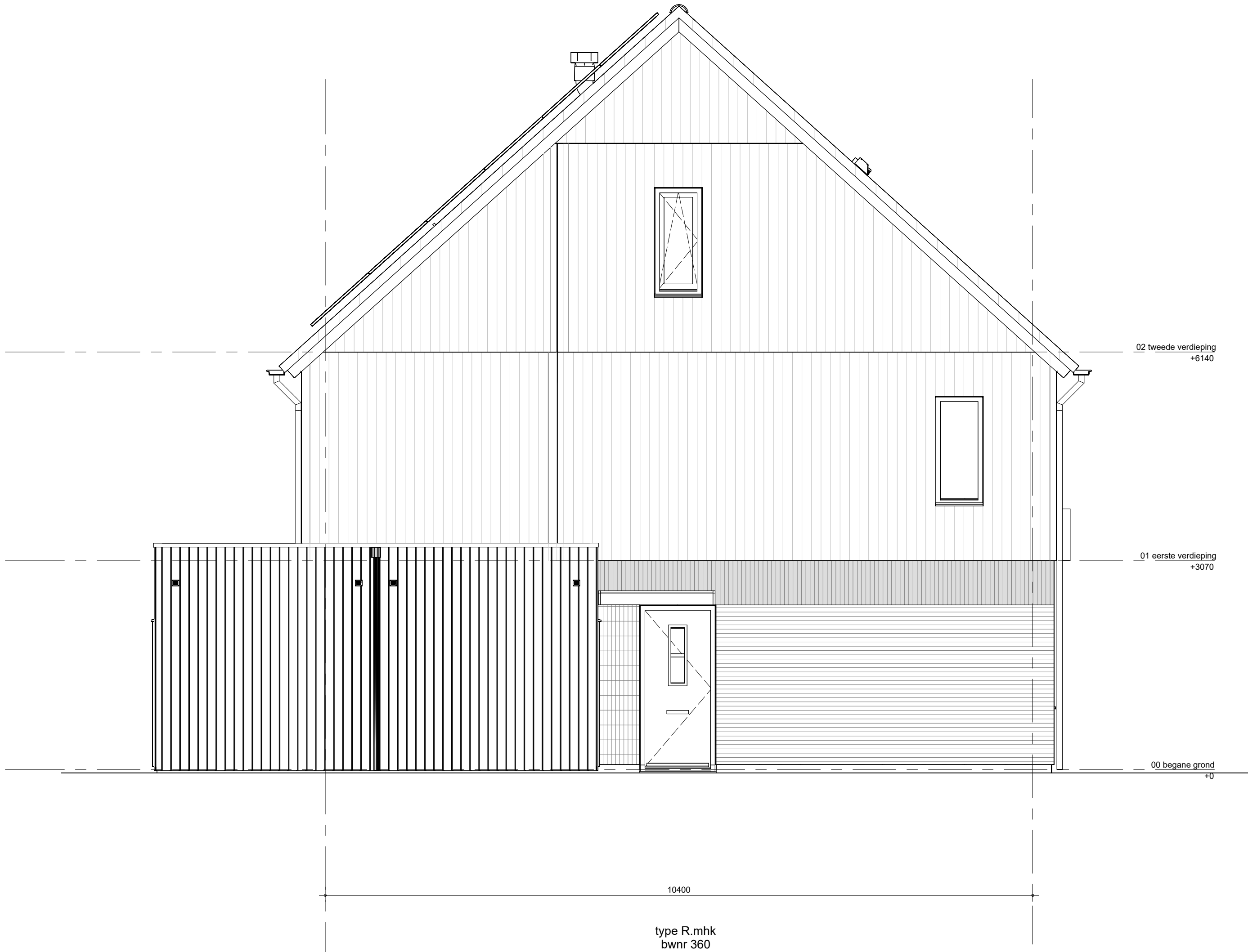
zijgevel links blok 10.3
