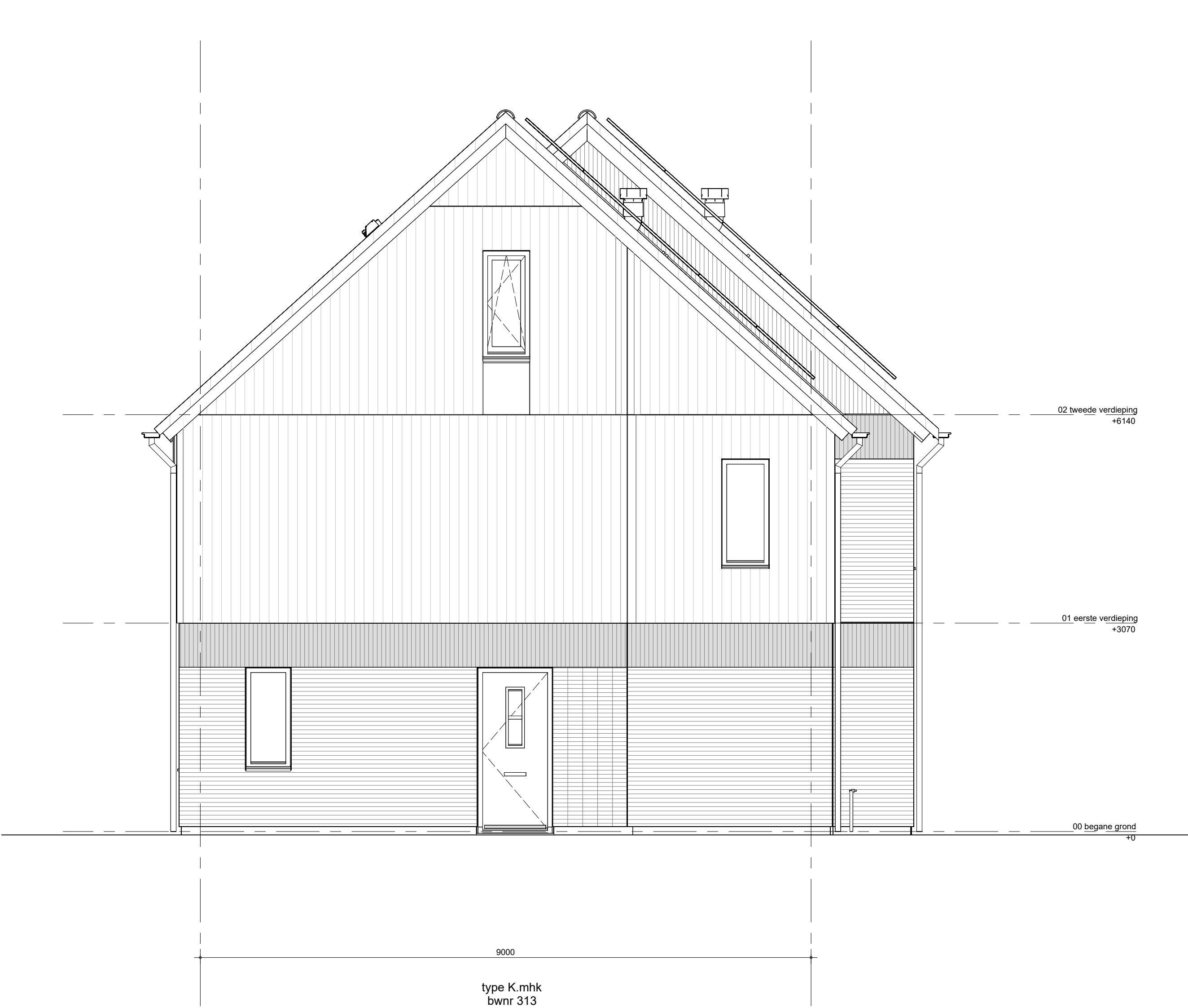
zijgevel rechts blok 03
