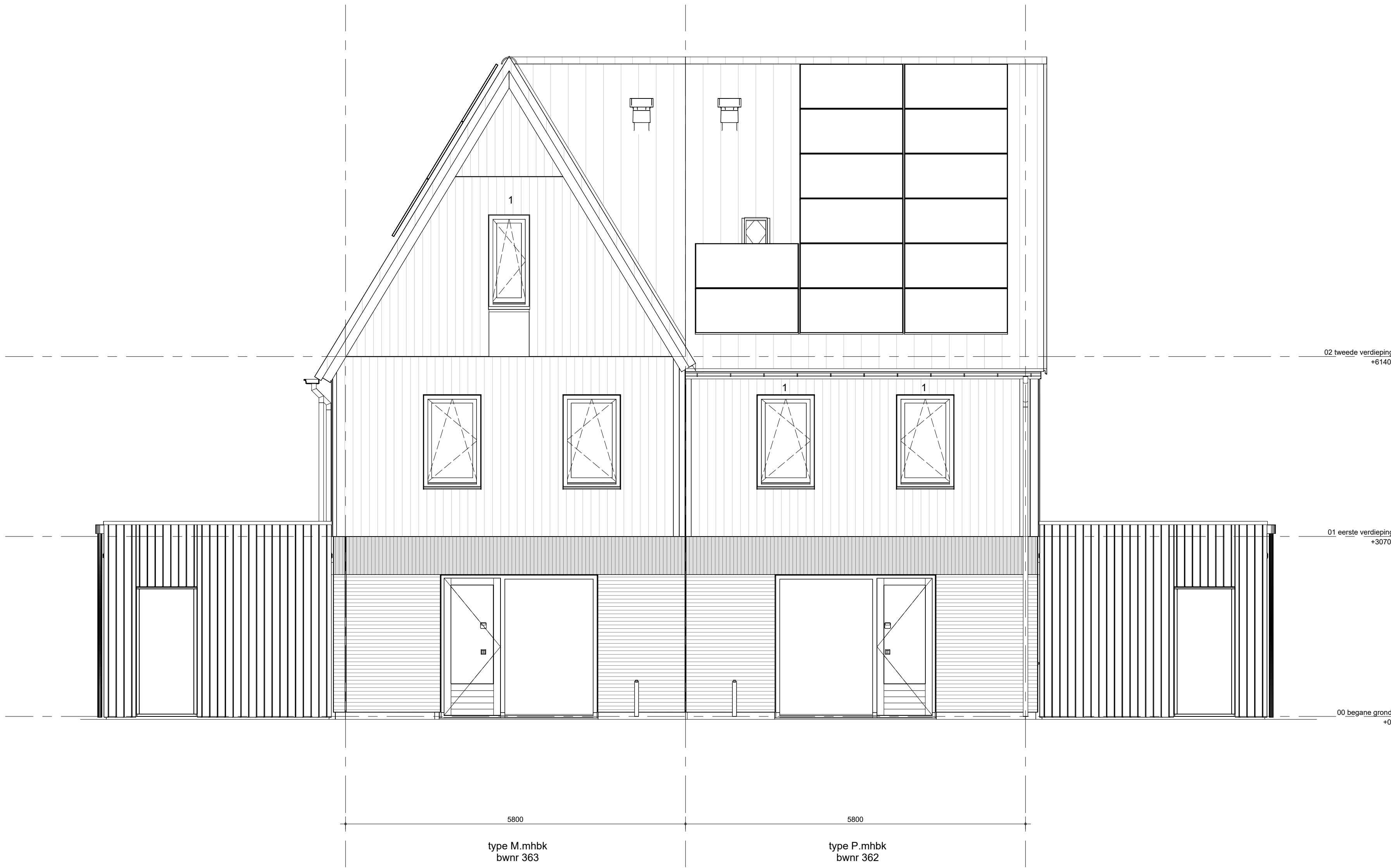
achtergevel blok 10.4
