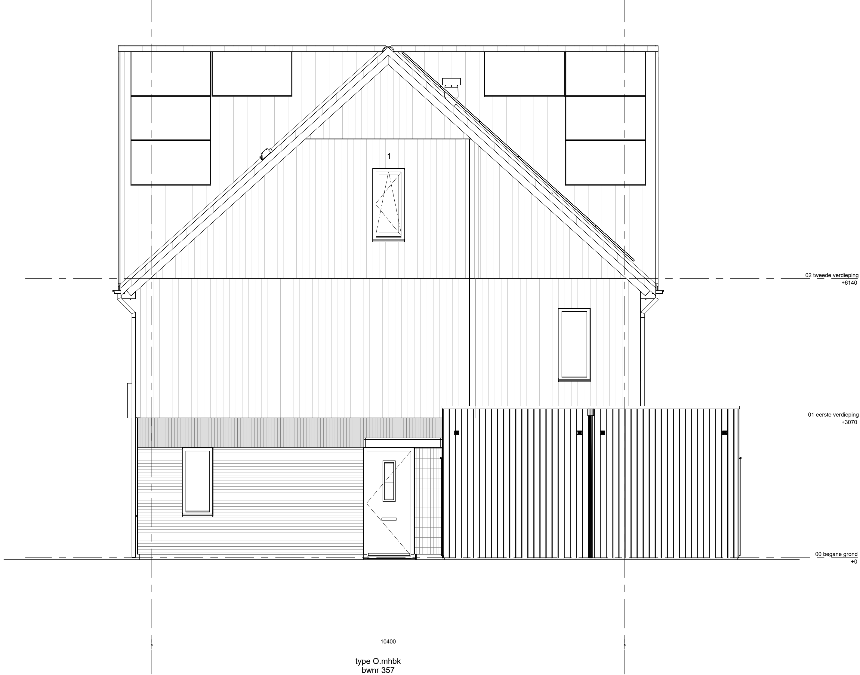
zijgevel rechts blok 10.1
