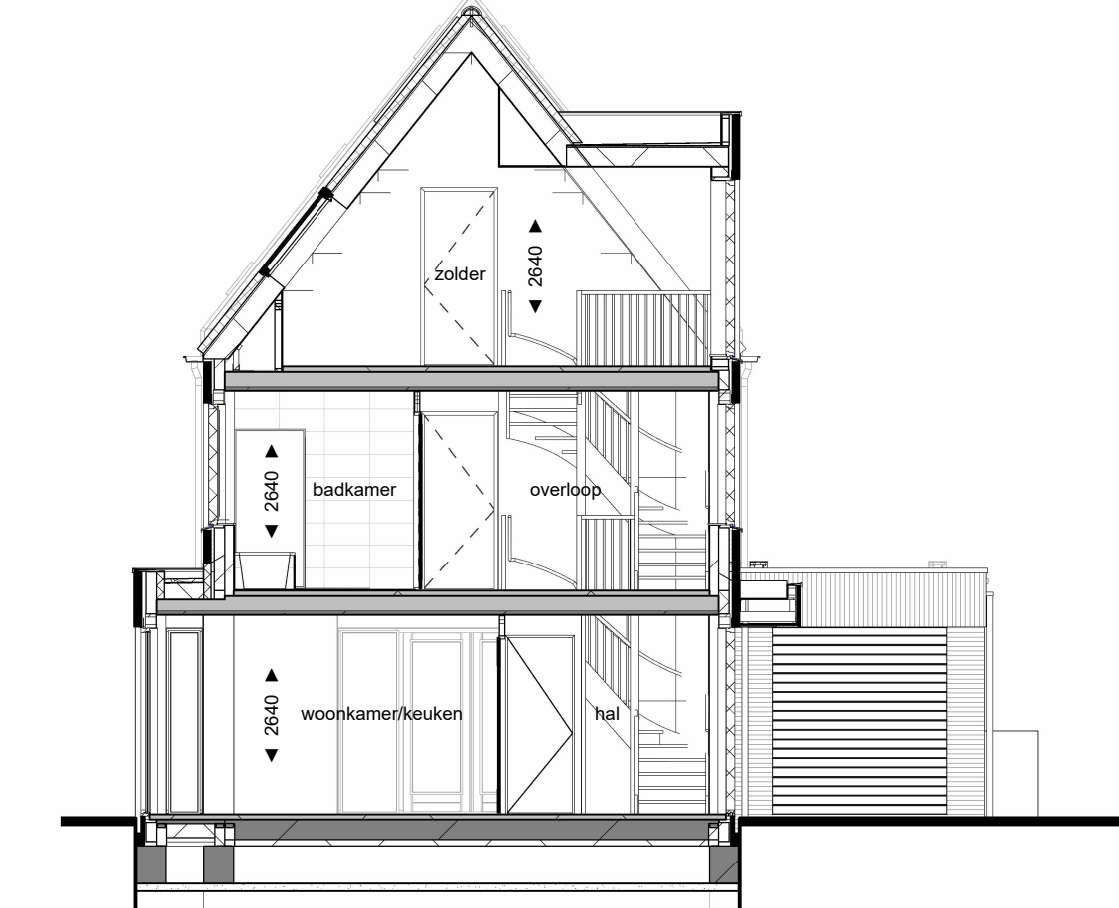
Doorsnede B-B
