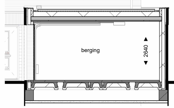
Doorsnede D-D
