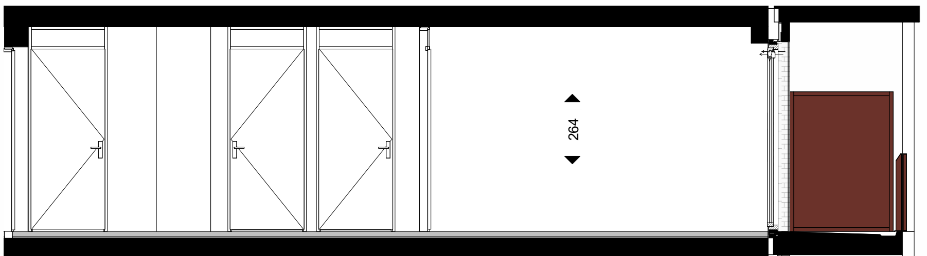
lengtedoorsnede 1:50
