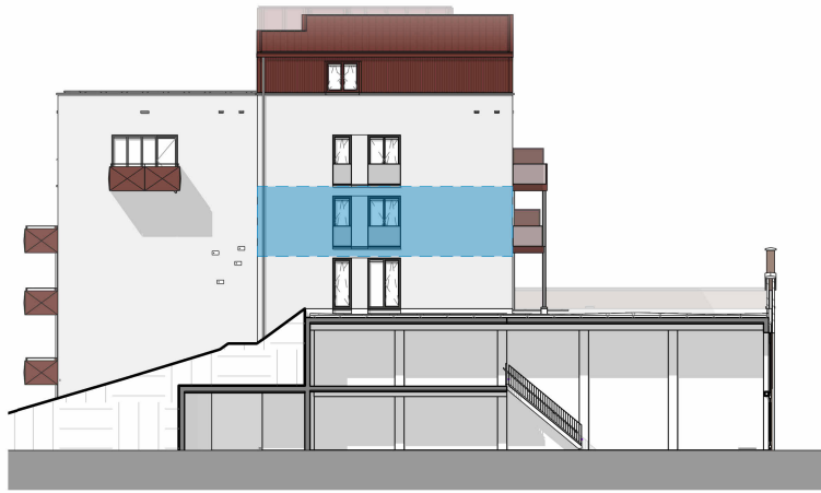
Zuidwestgevel 1:400
