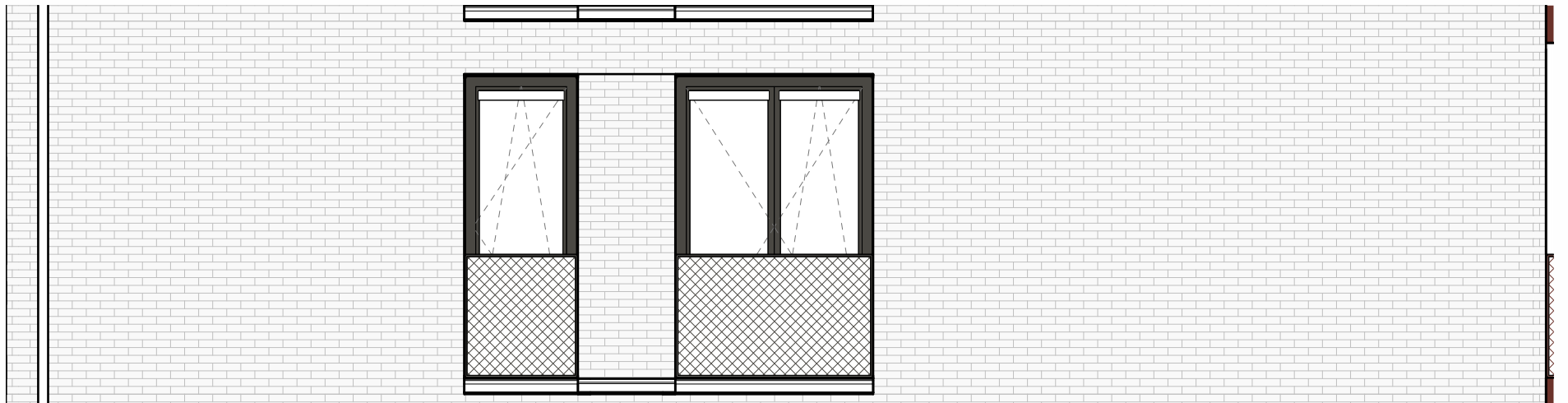
Gevelfragment Zuidwestgevel 1:50
