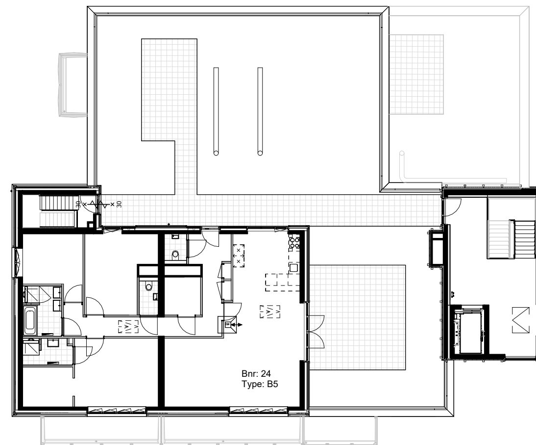
Vijfde verdieping 1:200
