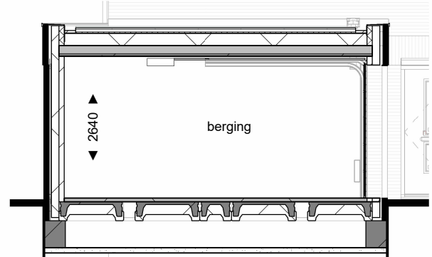
Doorsnede D-D
