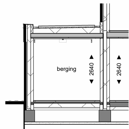
Doorsnede C-C
