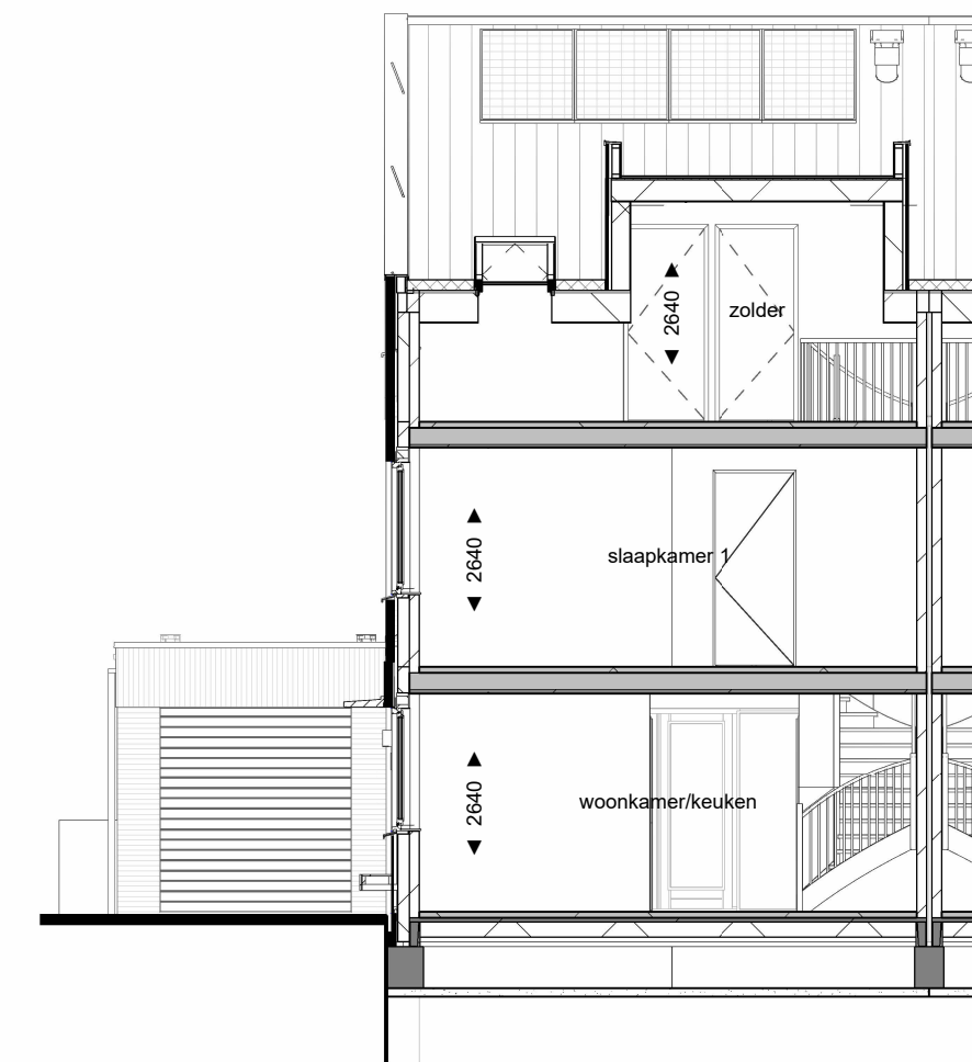
Doorsnede B-B
